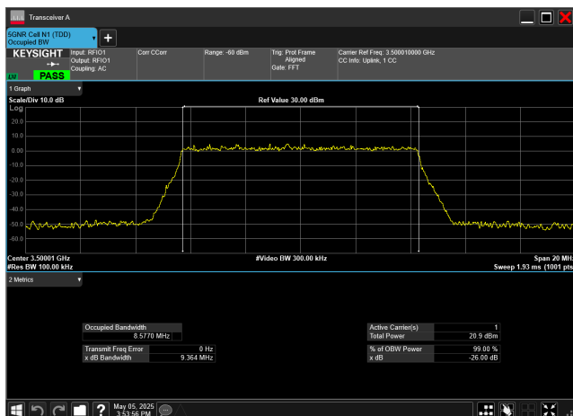
n78_1_10MHz_30kHz_3500MHz_DFT-s-OFDM QPSK_RB24@0
