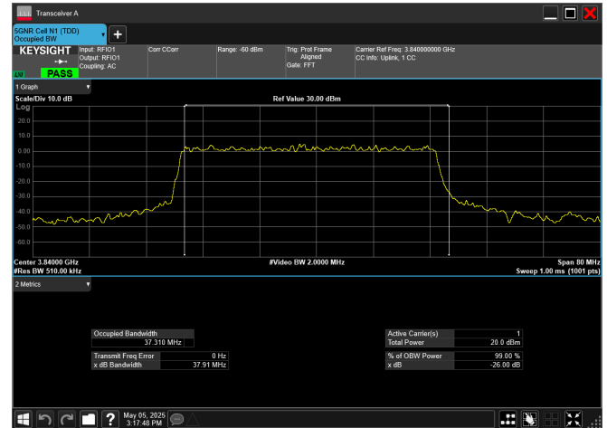
n77_3_40MHz_30kHz_3840MHz_CP-OFDM QPSK_RB106@0
