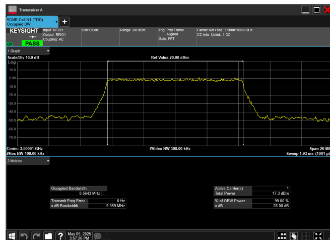
n78_1_10MHz_30kHz_3500MHz_CP-OFDM 16 QAM_RB24@0
