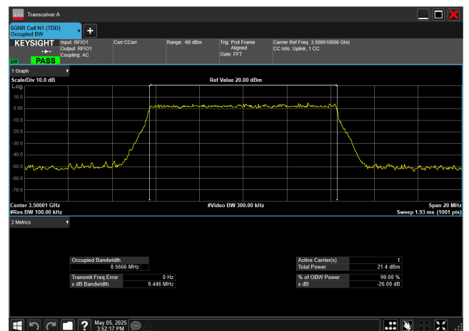
n78_1_10MHz_30kHz_3500MHz_DFT-s-OFDM 16 QAM_RB24@0
