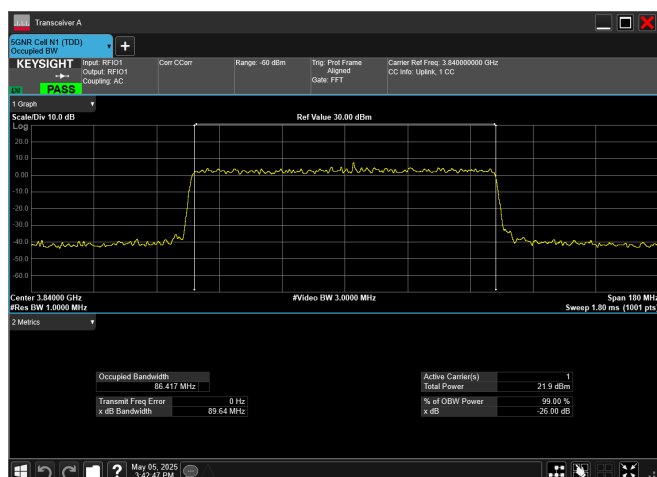
n77_3_90MHz_30kHz_3840MHz_DFT-s-OFDM QPSK_RB243@0
