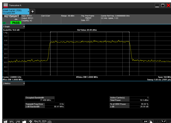
n77_3_90MHz_30kHz_3840MHz_DFT-s-OFDM QPSK_RB243@0
