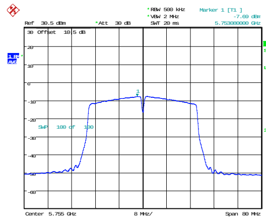
802.11n40_5755MHz
