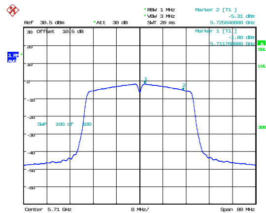
802.11n40_5710MHz
