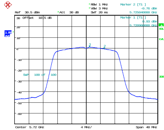
802.11n20_5720MHz
