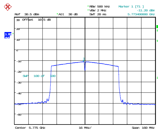
802.11ac80_5775MHz
