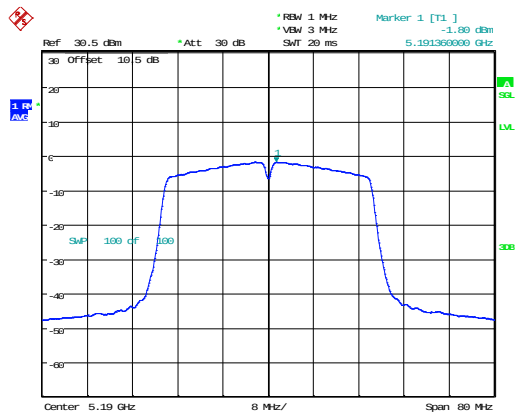
802.11n40_5190MHz
