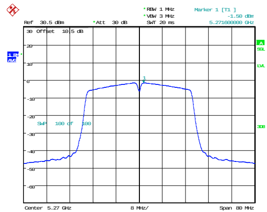
802.11n40_5270MHz
