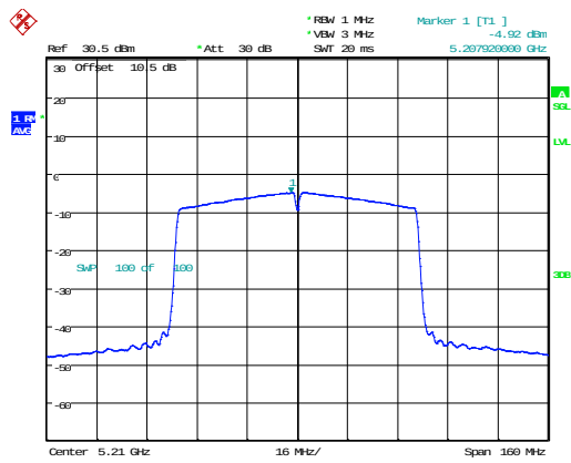
802.11ac80_5210MHz
