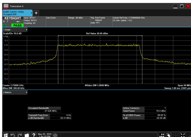
n78_3_30MHz_30kHz_3750MHz_CP-OFDM QPSK_RB78@0
