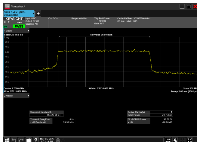
n78_3_100MHz_30kHz_3750MHz_DFT-s-OFDM 64 QAM_RB270@0
