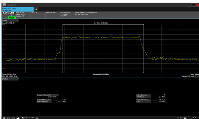
n78_3_70MHz_30kHz_3750MHz_DFT-s-OFDM QPSK_RB180@0
