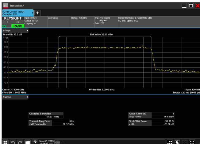
n78_3_70MHz_30kHz_3750MHz_DFT-s-OFDM QPSK_RB180@0
