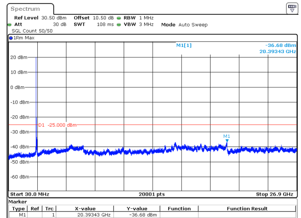
n41_100MHz_30kHz_2640MHz_DFT-s-OFDM QPSK_RB1@0 -36.68dBm
