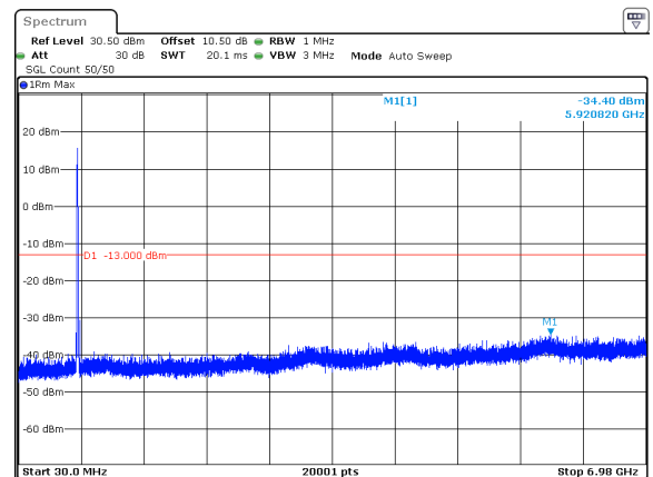
n71_10MHz_15kHz_680.5MHz_DFT-s-OFDM QPSK_RB50@0 -34.40dBm
