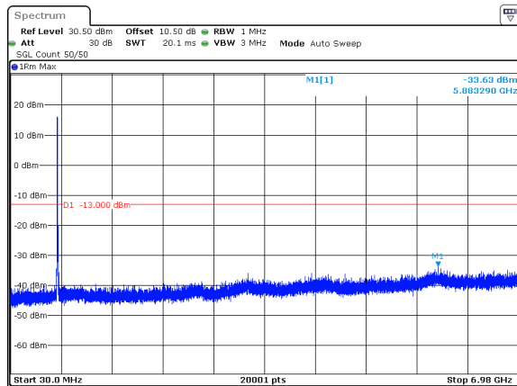
n71_10MHz_15kHz_668MHz_DFT-s-OFDM QPSK_RB50@0 -33.63dBm
