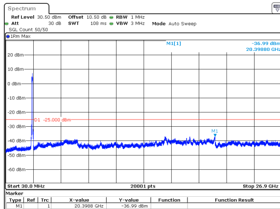
n41_100MHz_30kHz_2592.99MHz_DFT-s-OFDM QPSK_RB270@0 -36.99dBm
