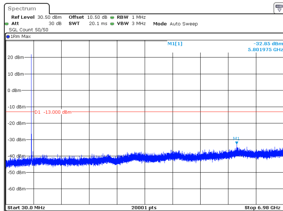
n71_10MHz_15kHz_668MHz_DFT-s-OFDM QPSK_RB1@0 -32.85dBm
