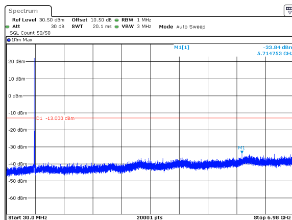
n71_10MHz_15kHz_693MHz_DFT-s-OFDM QPSK_RB1@51 -33.84dBm
