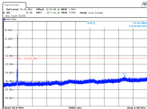
n71_10MHz_15kHz_693MHz_DFT-s-OFDM QPSK_RB50@0 -34.69dBm
