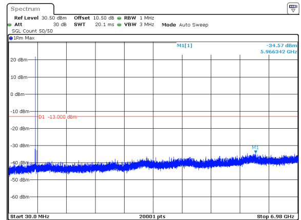
n71_10MHz_15kHz_668MHz_DFT-s-OFDM QPSK_RB1@51 -34.57dBm
