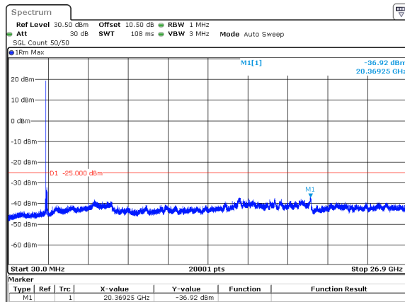
n41_100MHz_30kHz_2592.99MHz_DFT-s-OFDM QPSK_RB1@0 -36.92dBm
