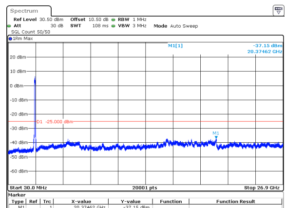
n41_100MHz_30kHz_2640MHz_DFT-s-OFDM QPSK_RB1@272 -36.47dBm n41_100MHz_30kHz_2640MHz_DFT-s-OFDM QPSK_RB270@0 -37.15dBm
