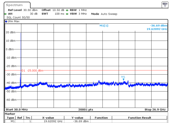
n41_100MHz_30kHz_2592.99MHz_DFT-s-OFDM QPSK_RB1@272 -36.69dBm
