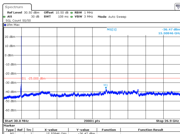
n41_100MHz_30kHz_2640MHz_DFT-s-OFDM QPSK_RB1@272 -36.47dBm n41_100MHz_30kHz_2640MHz_DFT-s-OFDM QPSK_RB270@0 -37.15dBm
