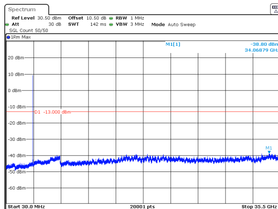
n77_1_20MHz_30kHz_3460MHz_DFT-s-OFDM QPSK_RB1@0 -38.80dBm
