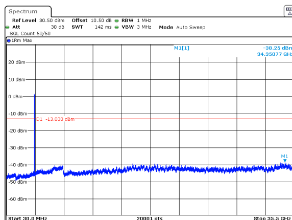
n78_1_20MHz_30kHz_3460MHz_DFT-s-OFDM QPSK_RB50@0 -38.25dBm
