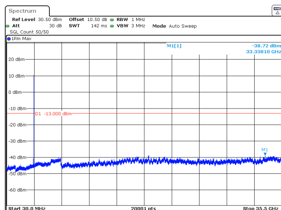
n78_1_20MHz_30kHz_3460MHz_DFT-s-OFDM QPSK_RB1@50 -38.72dBm
