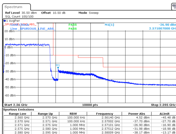
n7_10MHz_15kHz_2565MHz_DFT-s-OFDM QPSK_RB50@0
