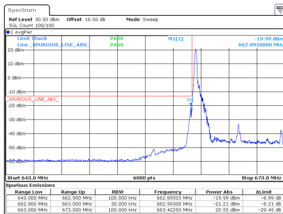
n71_10MHz_15kHz_668MHz_DFT-s-OFDM QPSK_RB1@0
