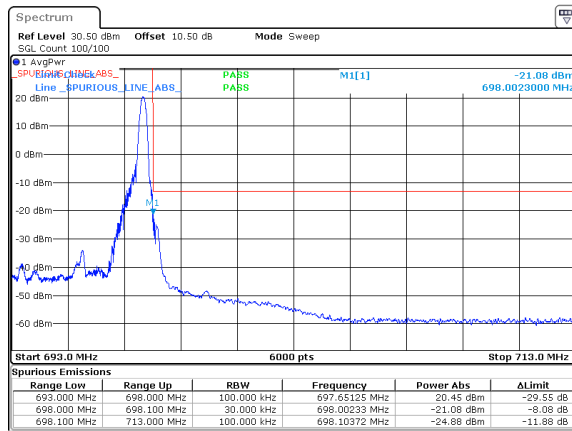
n71_5MHz_15kHz_695.5MHz_DFT-s-OFDM QPSK_RB1@24
