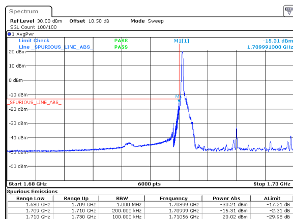
n66_20MHz_15kHz_1720MHz_DFT-s-OFDM QPSK_RB1@0
