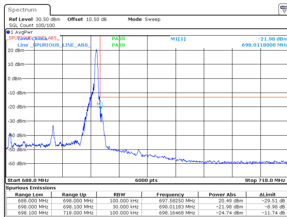
n71_10MHz_15kHz_693MHz_DFT-s-OFDM QPSK_RB1@51
