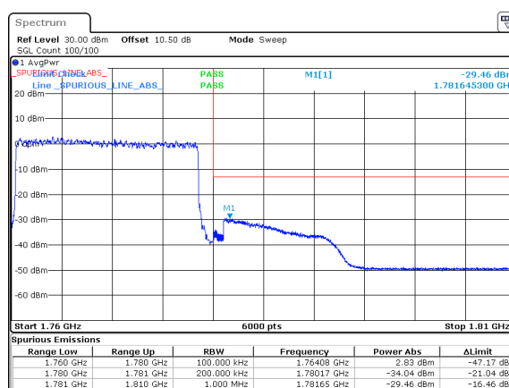
n66_20MHz_15kHz_1770MHz_DFT-s-OFDM QPSK_RB100@0
