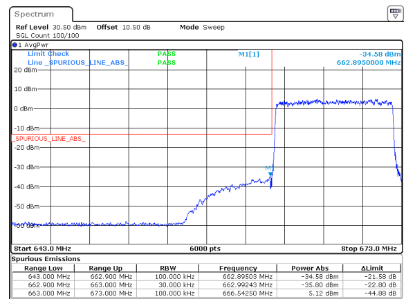
n71_10MHz_15kHz_668MHz_DFT-s-OFDM QPSK_RB50@0
