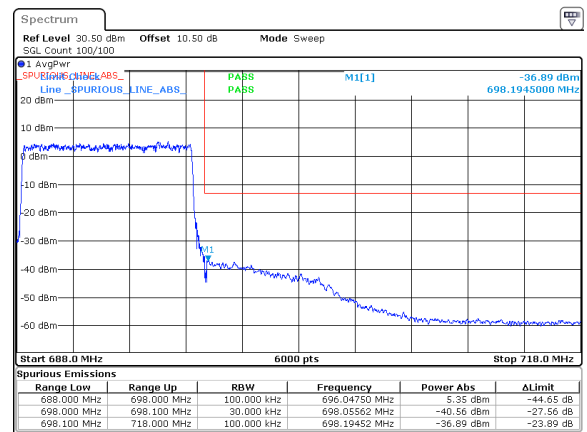
n71_10MHz_15kHz_693MHz_DFT-s-OFDM QPSK_RB50@0
