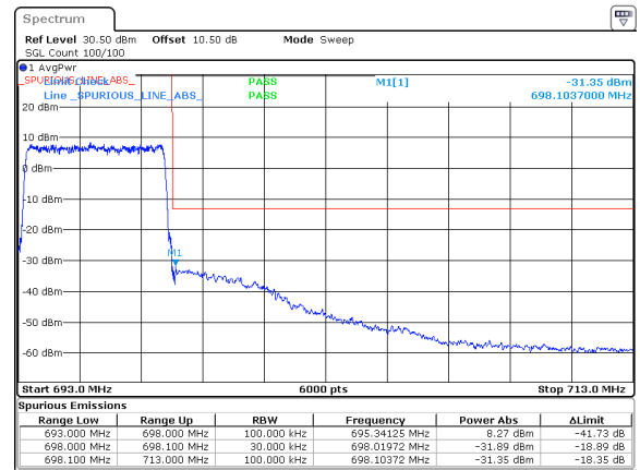
n71_5MHz_15kHz_695.5MHz_DFT-s-OFDM QPSK_RB25@0
