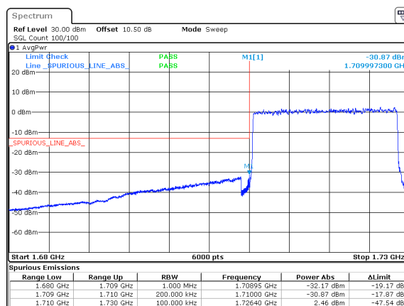
n66_20MHz_15kHz_1720MHz_DFT-s-OFDM QPSK_RB100@0
