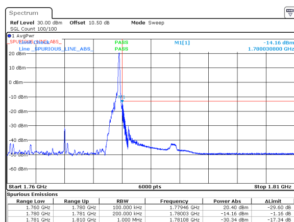
n66_20MHz_15kHz_1770MHz_DFT-s-OFDM QPSK_RB1@105
