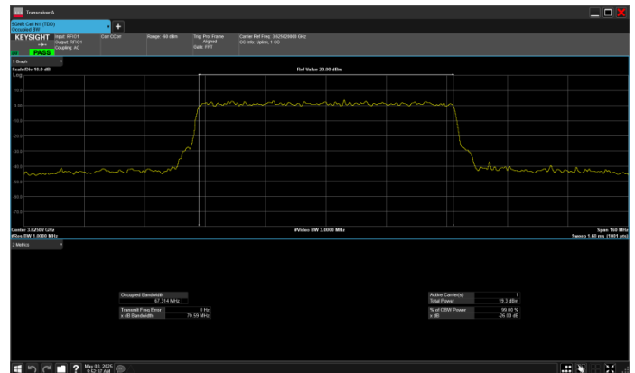
n78_2_80MHz_30kHz_3625MHz_DFT-s-OFDM \pi/2 BPSK_RB216@0
