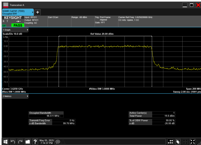
n78_2_100MHz_30kHz_3625MHz_CP-OFDM QPSK_RB273@0
