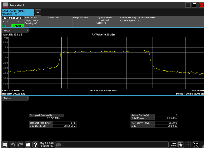
n78_2_30MHz_30kHz_3625MHz_DFT-s-OFDM 16 QAM_RB75@0
