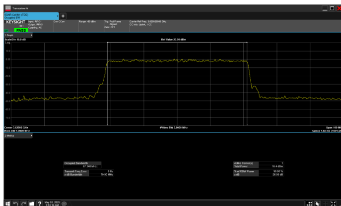
n78_2_80MHz_30kHz_3625MHz_DFT-s-OFDM QPSK_RB216@0
