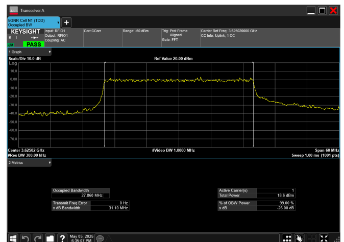
n78_2_30MHz_30kHz_3625MHz_CP-OFDM QPSK_RB78@0
