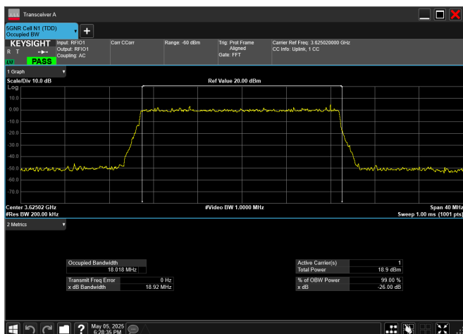
n78_2_20MHz_30kHz_3625MHz_CP-OFDM QPSK_RB51@0
