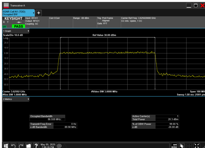
n78_2_90MHz_30kHz_3625MHz_DFT-s-OFDM 256 QAM_RB243@0
