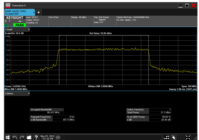
n78_2_90MHz_30kHz_3625MHz_DFT-s-OFDM 64 QAM_RB243@0
