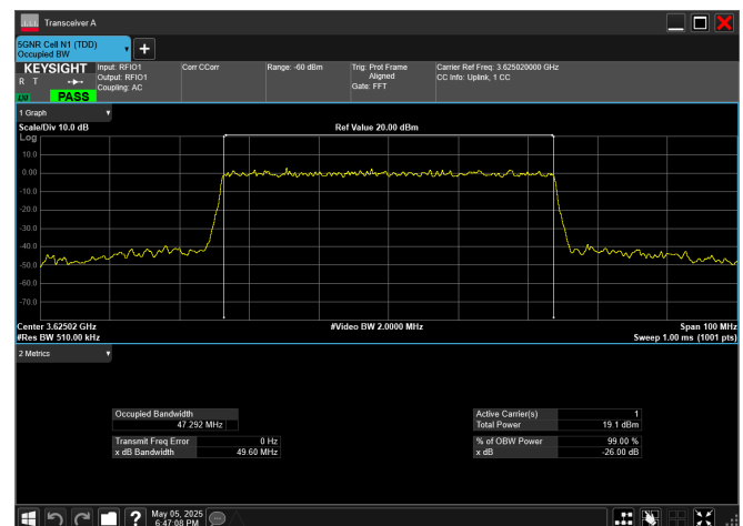
n78_2_50MHz_30kHz_3625MHz_CP-OFDM QPSK_RB133@0
