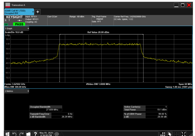
n78_2_30MHz_30kHz_3625MHz_DFT-s-OFDM 64 QAM_RB75@0
