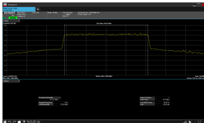
n78_2_70MHz_30kHz_3625MHz_CP-OFDM QPSK_RB189@0
