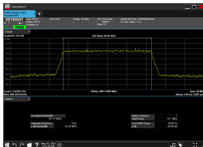
n78_2_20MHz_30kHz_3625MHz_CP-OFDM 256 QAM_RB51@0
