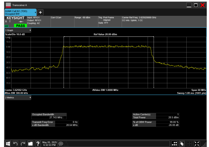
n78_2_30MHz_30kHz_3625MHz_DFT-s-OFDM 64 QAM_RB75@0
