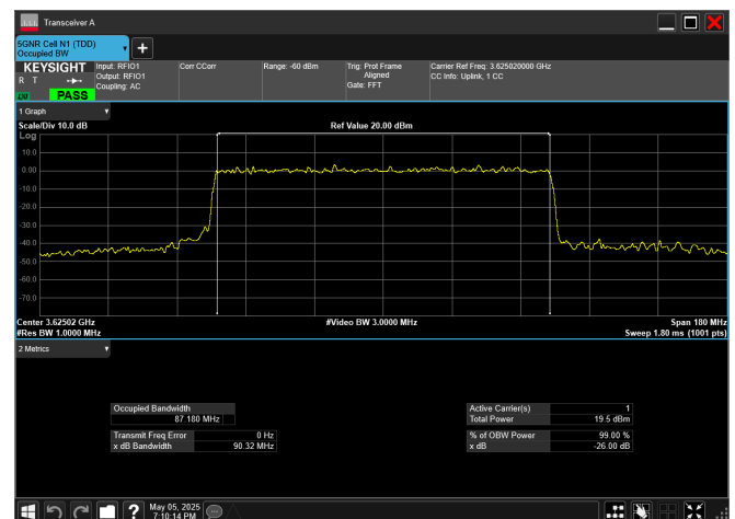
n78_2_90MHz_30kHz_3625MHz_CP-OFDM QPSK_RB245@0
