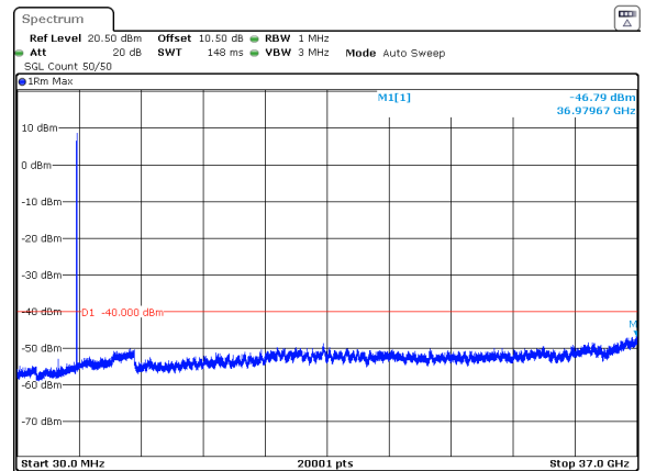
n78_2_15MHz_30kHz_3557.5MHz_DFT-s-OFDM QPSK_RB1@37 -46.79dBm
