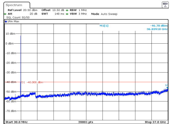
n78_2_15MHz_30kHz_3625MHz_DFT-s-OFDM QPSK_RB1@0 -46.78dBm
