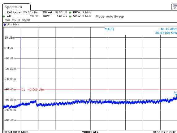
n78_2_15MHz_30kHz_3625MHz_DFT-s-OFDM QPSK_RB1@37 -46.42dBm n78_2_15MHz_30kHz_3625MHz_DFT-s-OFDM QPSK_RB36@0 -46.56dBm
