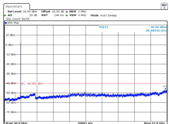
n78_2_15MHz_30kHz_3625MHz_DFT-s-OFDM QPSK_RB1@37 -46.42dBm n78_2_15MHz_30kHz_3625MHz_DFT-s-OFDM QPSK_RB36@0 -46.56dBm
