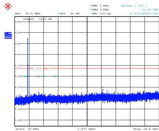
20MHz_Low_QPSK_1@0(30MHz~18.8GHz)
