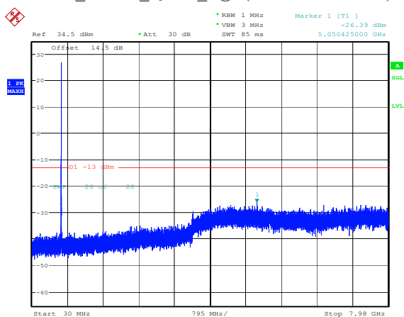
10MHz_Middle_QPSK_1@0(30MHz~7.98GHz)
