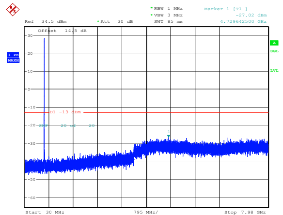
10MHz_Low_QPSK_1@0(30MHz~7.98GHz)
