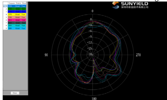
DCS1800 WCDMA: 4 LTE B3/B4 \Phi=90^\circ
