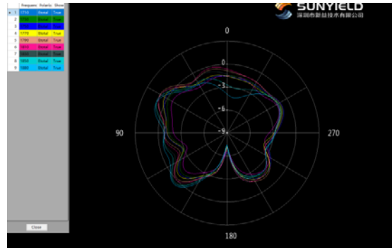
DCS1800 WCDMA: 4 LTE B3/B4 \Phi=0^\circ
