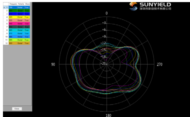
GSM850 / WCDMA B5 / LTE B5/B20 Phi=0deg
