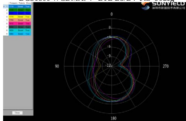
DCS1800 WCDMA: 4 LTE B3/B4 \Theta=90^\circ
