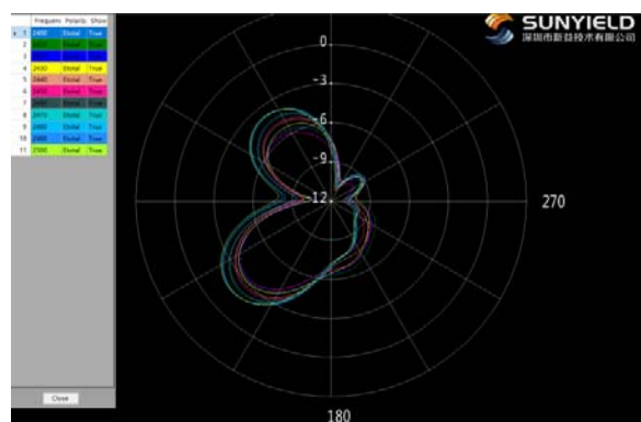
BT/ 2.4G WIFI Theta=90deg
