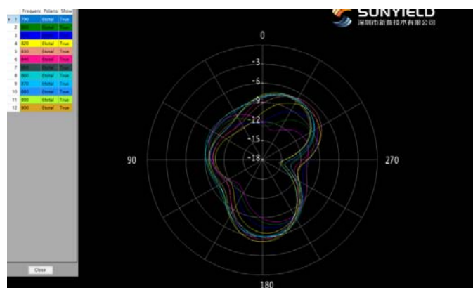
GSM850 / WCDMA B5 / LTE B5/B20 Theta=90deg
