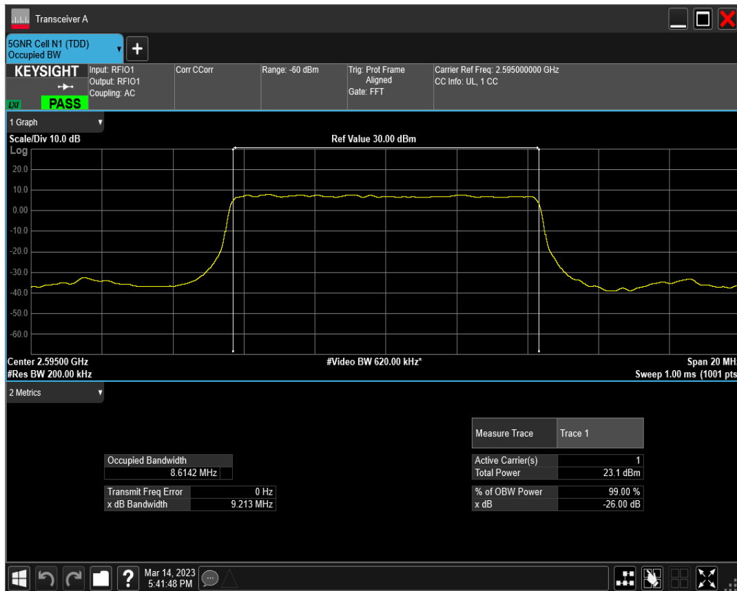
n38 SCS=30kHz DFT_QPSK BW=10MHz Channel=519000 RB=24@0
