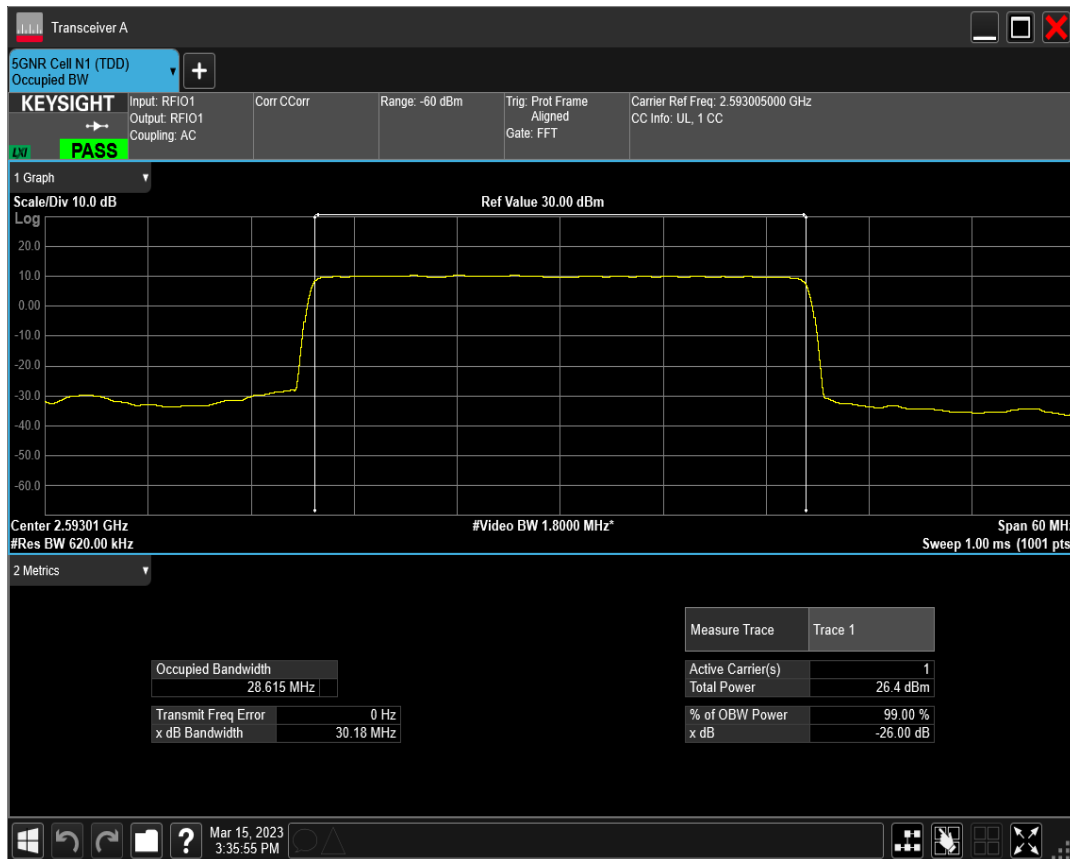
n41 SCS=15kHz DFT_QPSK BW=30MHz Channel=518601 RB=160@0
