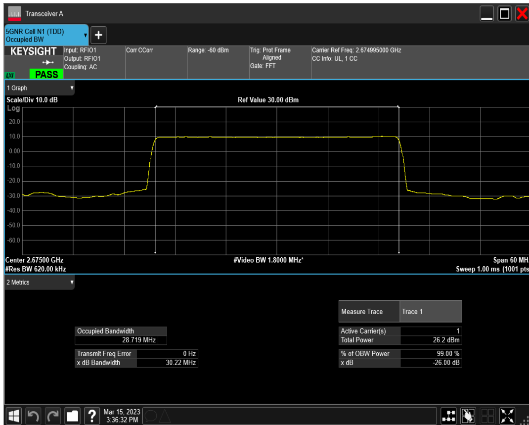
n41 SCS=15kHz DFT_QPSK BW=30MHz Channel=534999 RB=160@0
