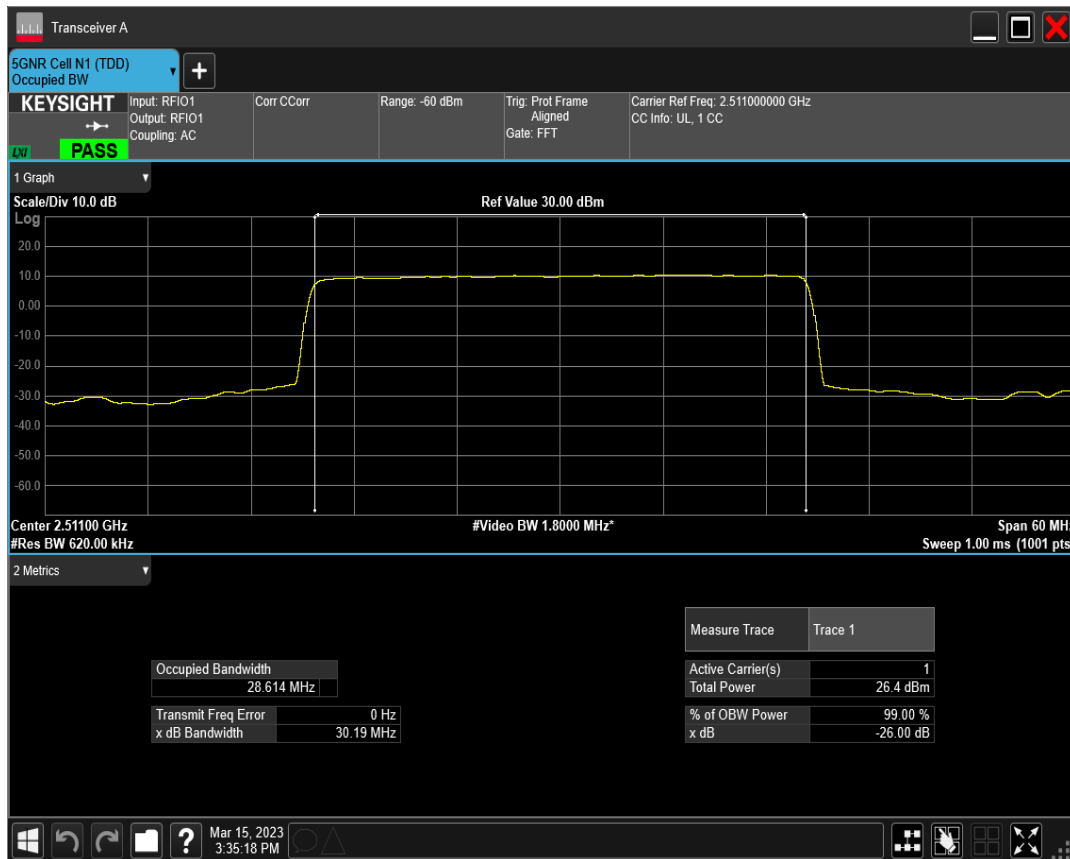
n41 SCS=15kHz DFT_QPSK BW=30MHz Channel=502200 RB=160@0
