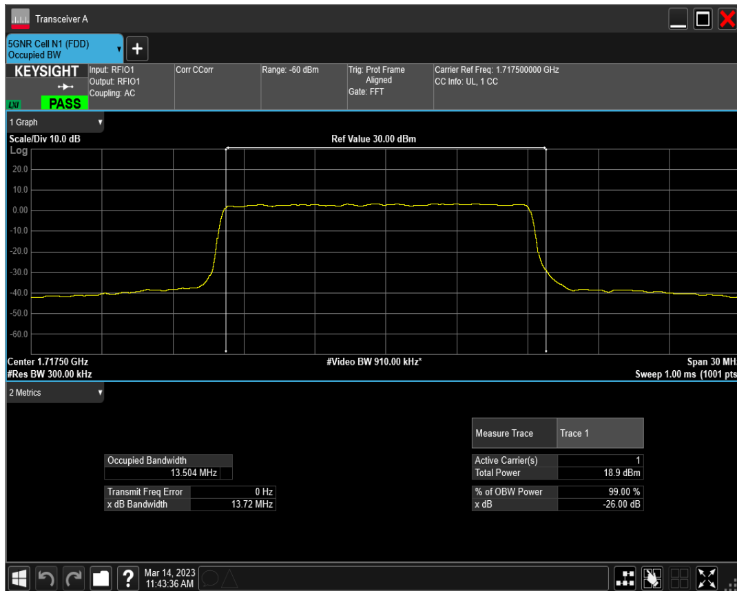
n66 SCS=30kHz CP_QPSK BW=15MHz Channel=343500 RB=38@0
