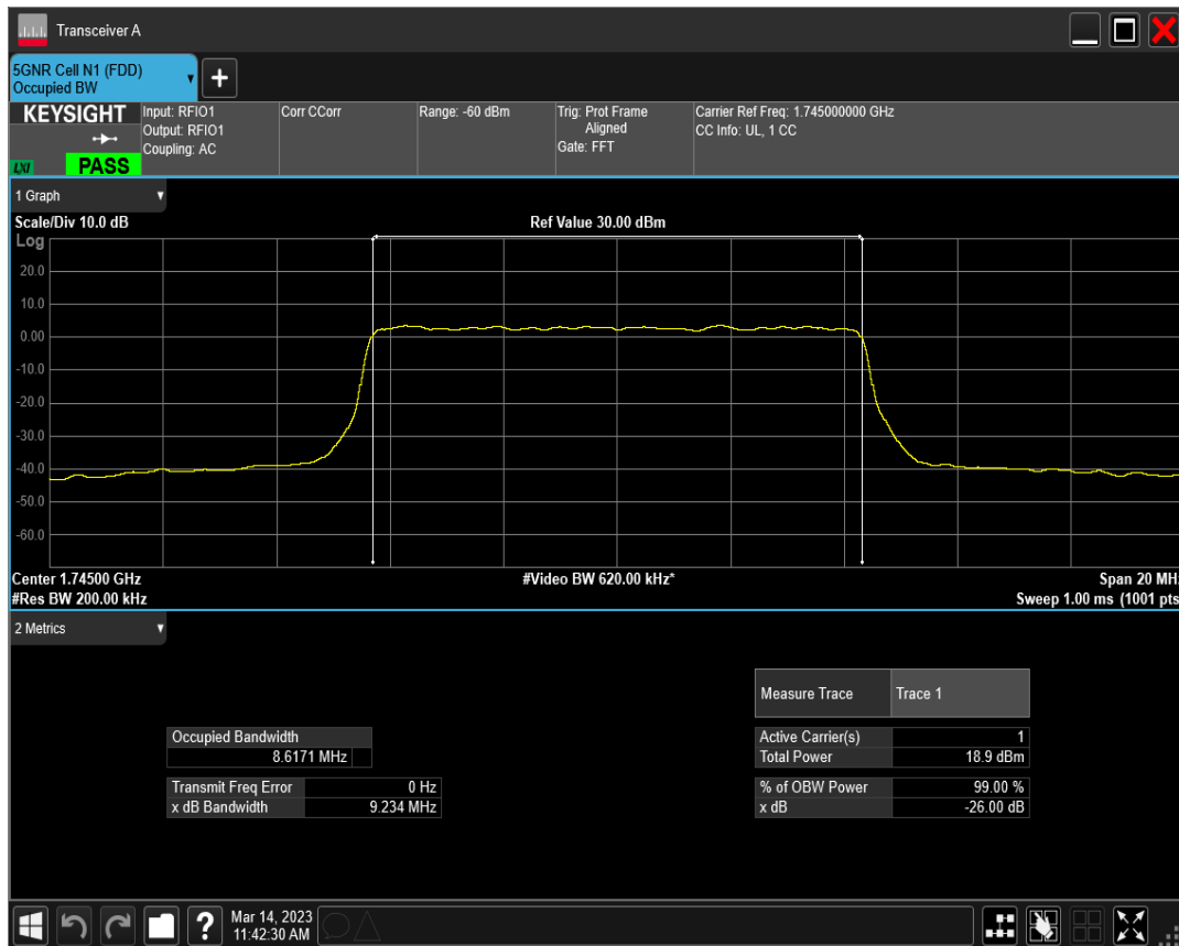
n66 SCS=30kHz CP_QPSK BW=10MHz Channel=349000 RB=24@0
