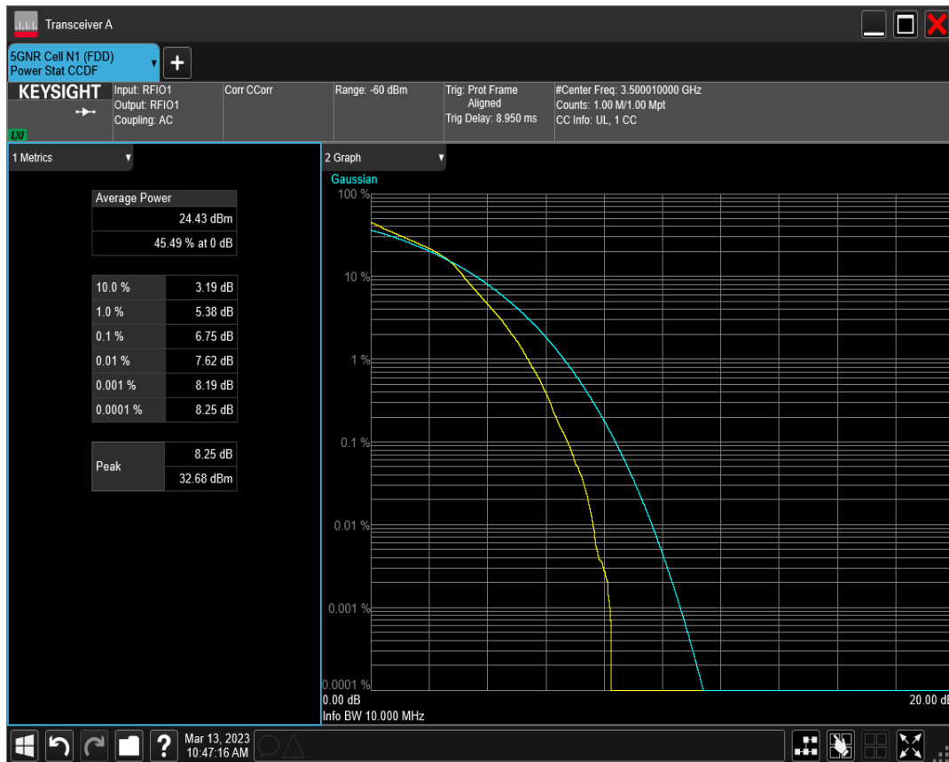
n77(3450-3550) SCS=15kHz DFT_QAM64 BW=10MHz Channel=633334 RB=50@0
