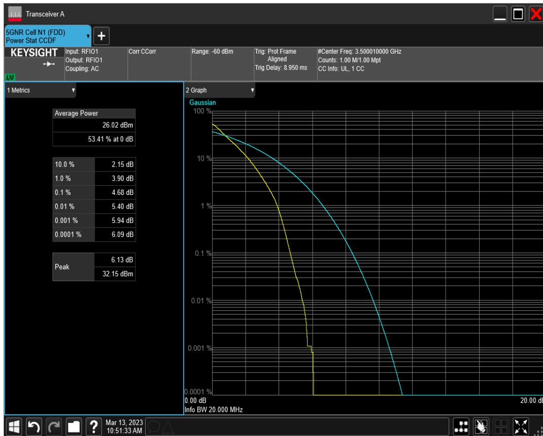
n77(3450-3550) SCS=15kHz DFT_QPSK BW=20MHz Channel=633334 RB=100@0
