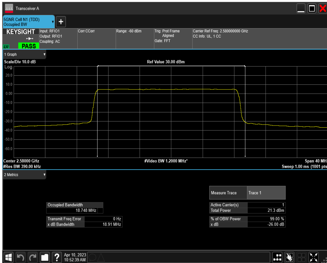
n38 SCS=15kHz DFT_QAM256 BW=20MHz Channel=516000 RB=100@0
