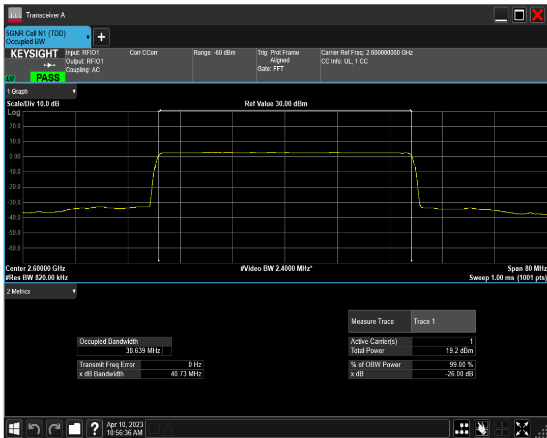
n38 SCS=15kHz CP_QPSK BW=40MHz Channel=520000 RB=216@0
