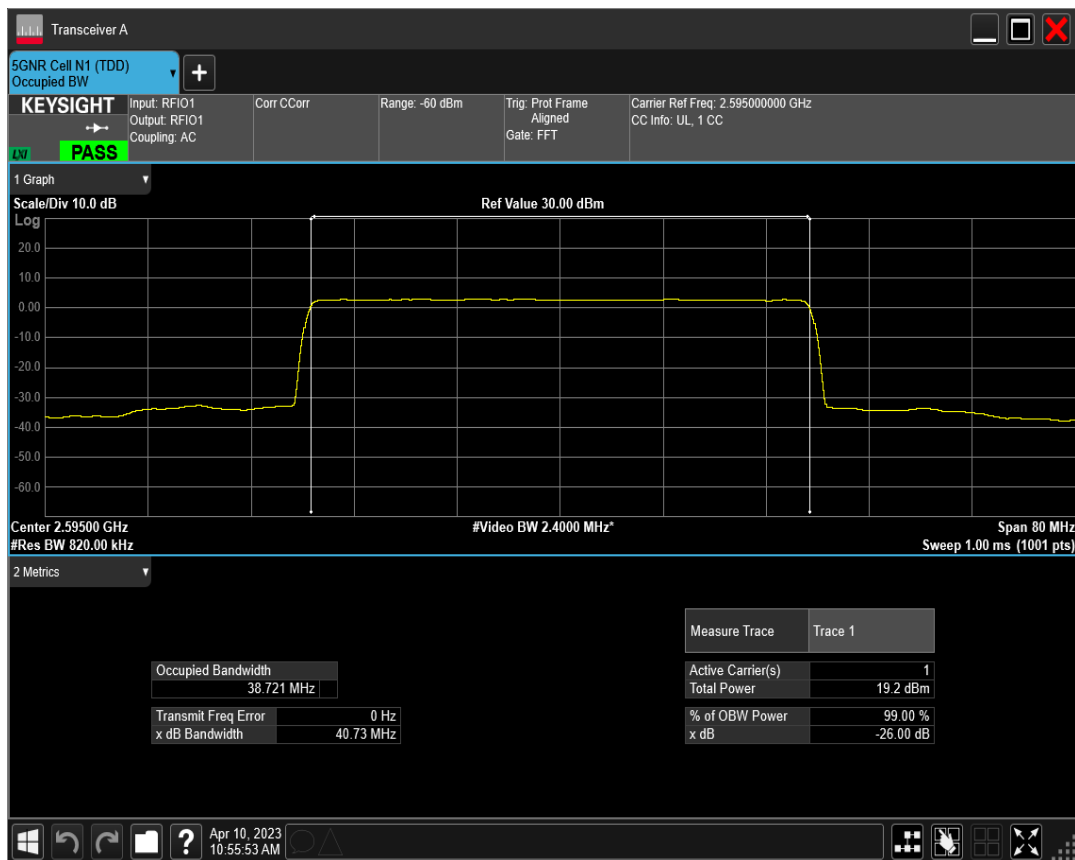
n38 SCS=15kHz CP_QPSK BW=40MHz Channel=519000 RB=216@0
