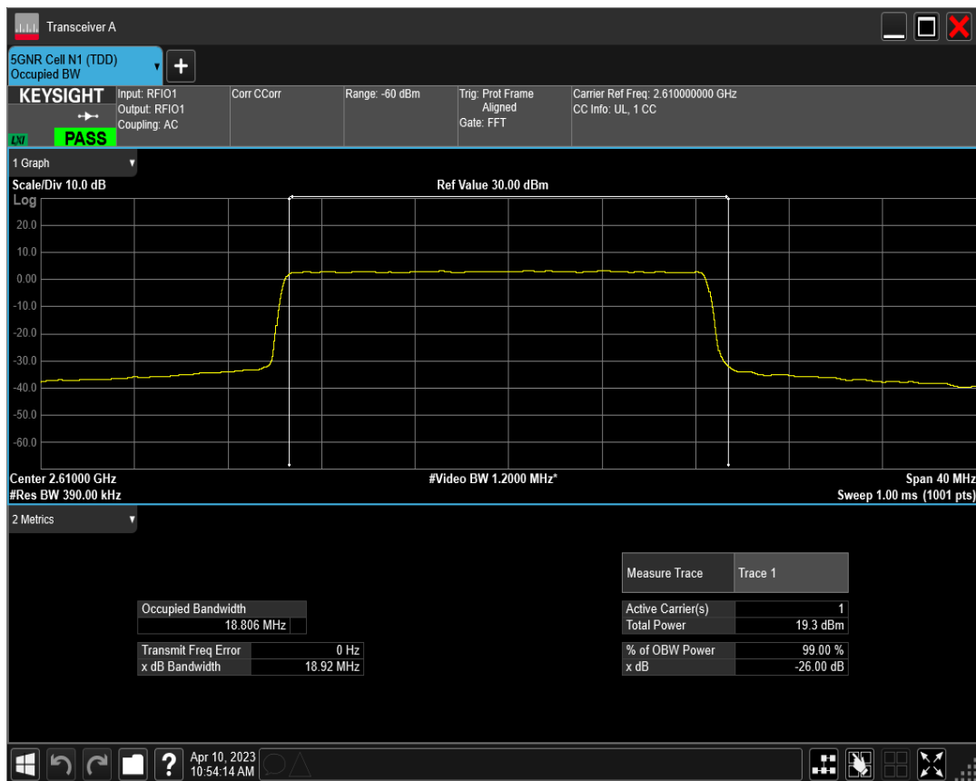
n38 SCS=15kHz CP_QPSK BW=20MHz Channel=522000 RB=106@0
