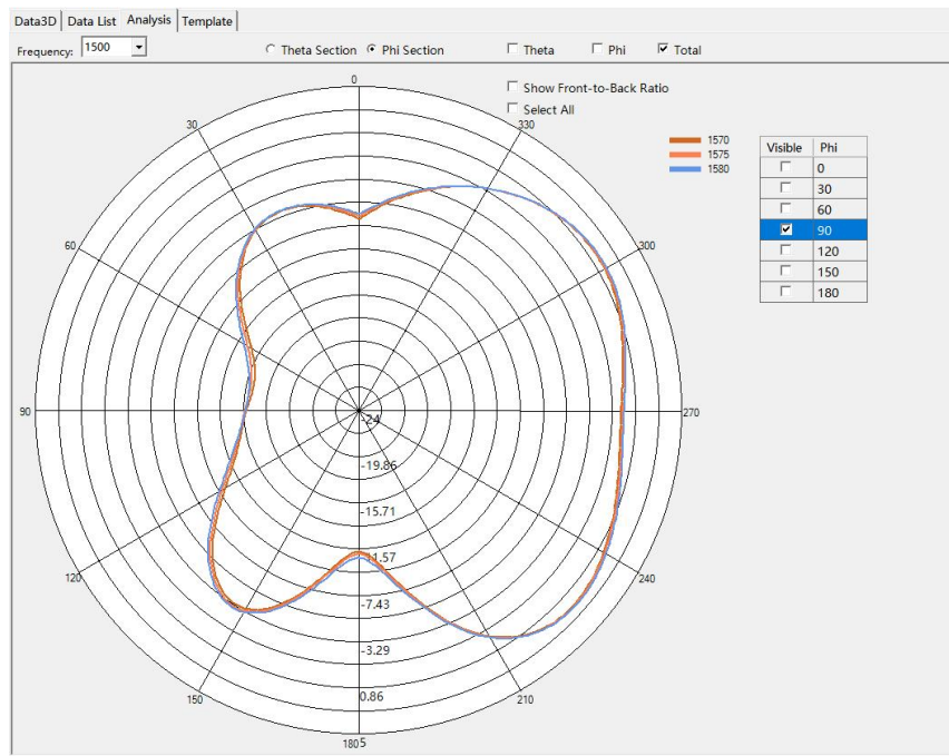
GPS Phi=90deg
