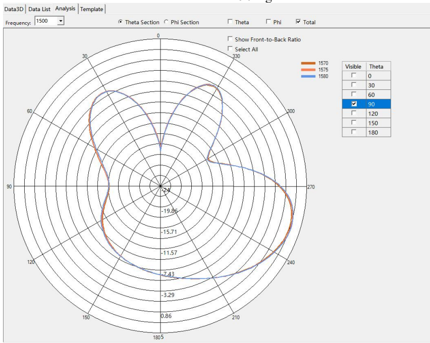
GPS Theta=90deg
