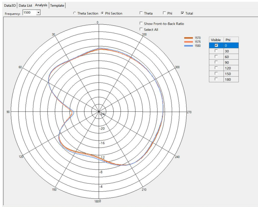
GPS Phi=0deg
