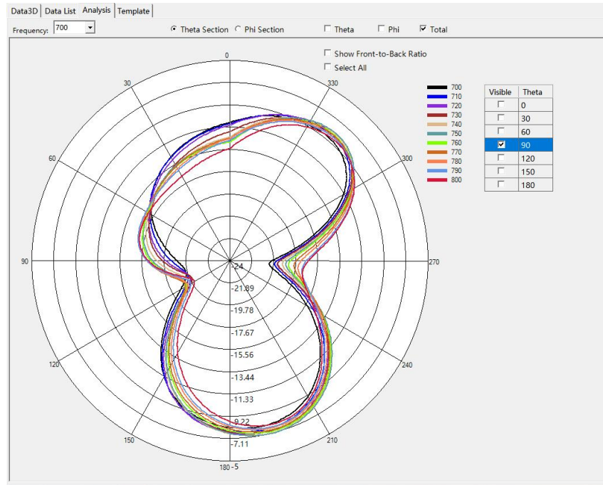
LTE B28 Theta=90deg
