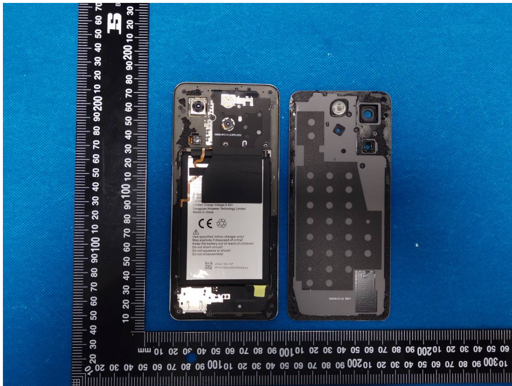
NFC ANT
