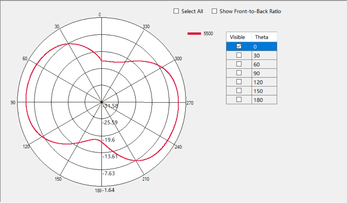
5G Phi=0deg
