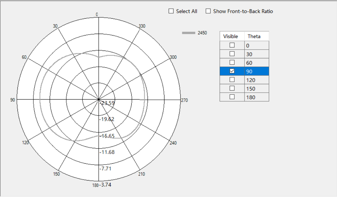
2.4G Theta=90deg
