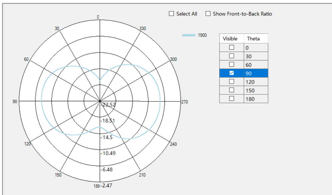
LTE B2 G1900 W2 Theta=90deg
