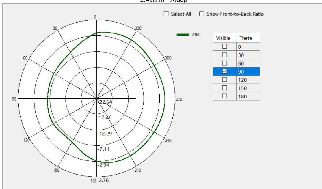
2.4G Theta=90deg
