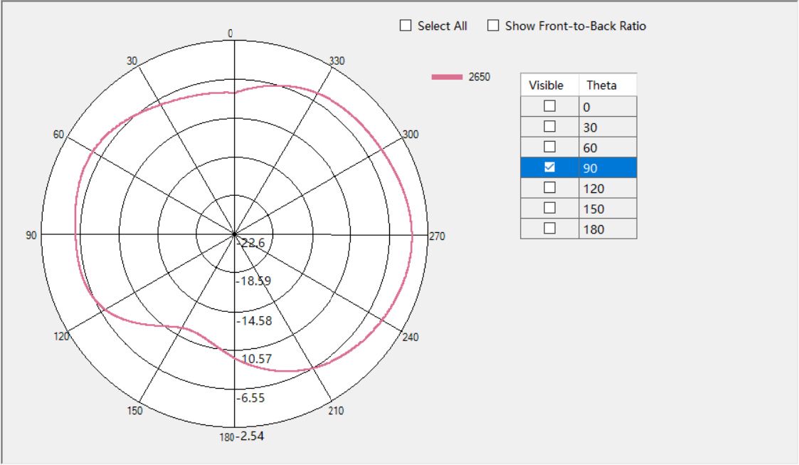
LTE B41 Theta=90deg
