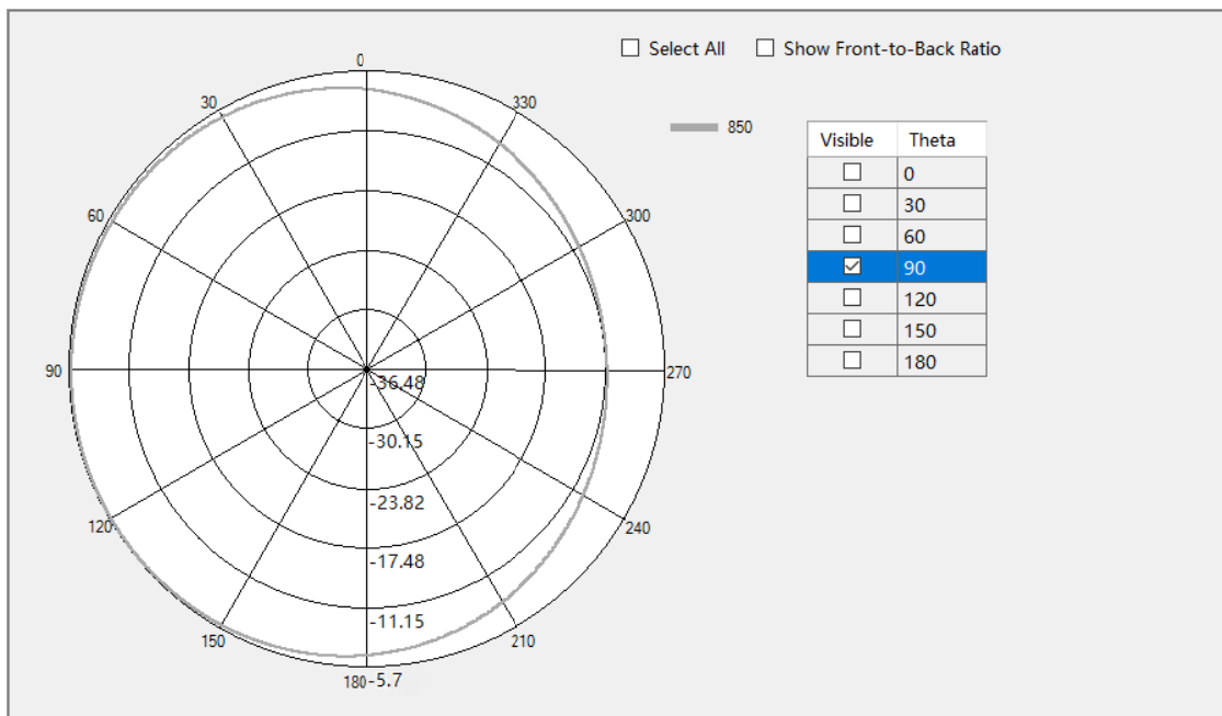
GSM850 / WCDMA B5 / LTE B5/B20 Theta=90deg
