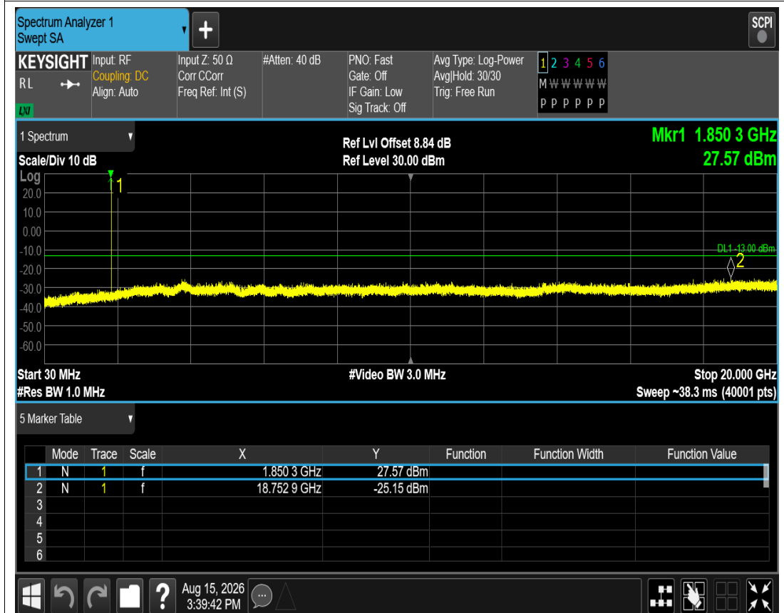
EGPRS1900 Channel=512
