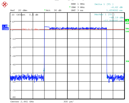
3DH3_Hopping 1.659ms
