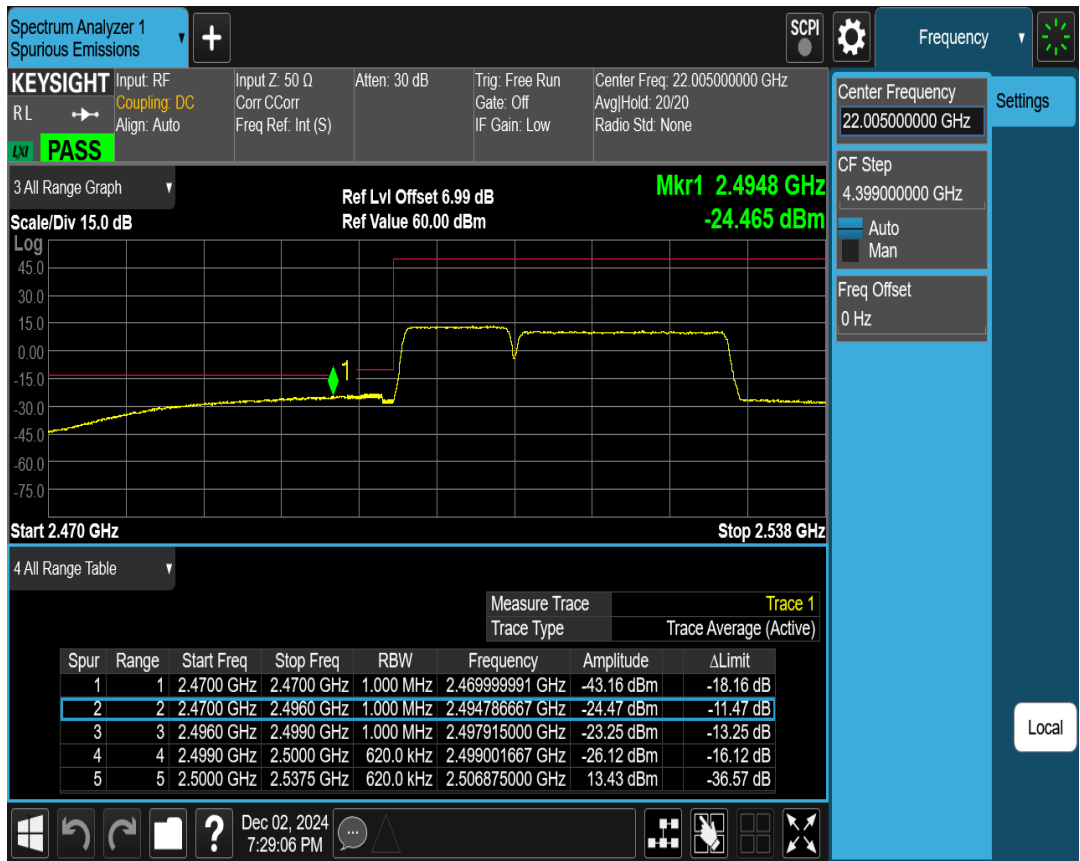
7C 16QAM PCC BW=10MHz Ch=2805 RB=1@0,SCC BW=20MHz Ch=2949 RB=1@99
