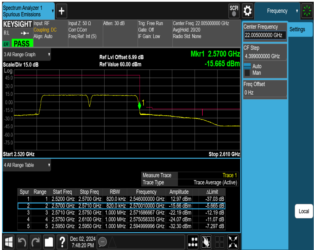
7C 16QAM PCC BW=20MHz Ch=3152 RB=1@0,SCC BW=20MHz Ch=3350 RB=1@99
