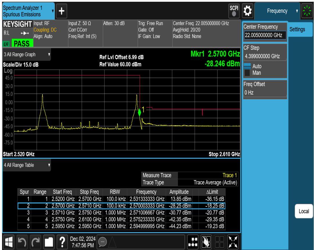
7C 16QAM PCC BW=20MHz Ch=3201 RB=100@0,SCC BW=15MHz Ch=3372 RB=75@0
