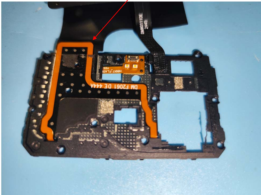
NFC ANT
