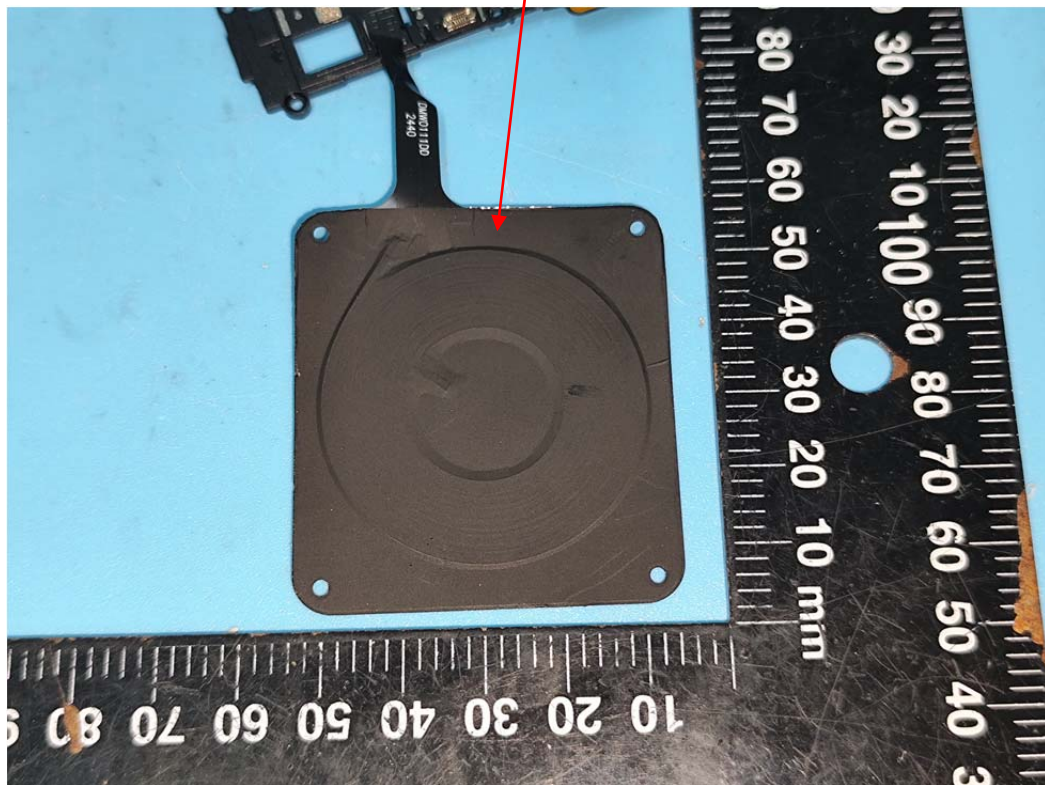
WPT ANT
