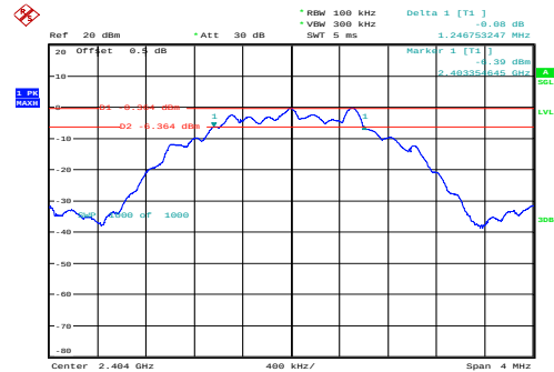
Low 1.247MHz
