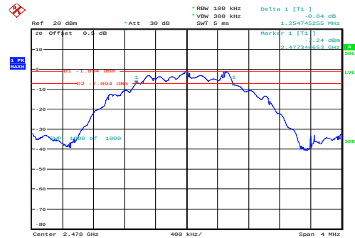
High 1.255MHz
