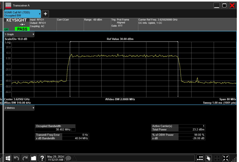
40MHz_15kHz_3625MHz_DFT-s-OFDM QPSK_RB216@0
