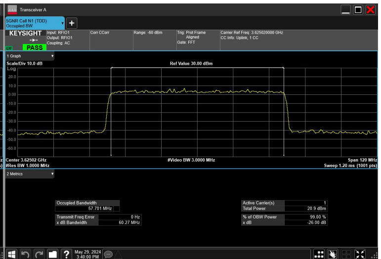
60MHz_30kHz_3625MHz_CP-OFDM QPSK_RB162@0
