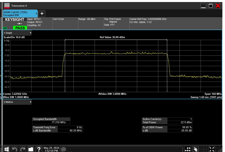
80MHz_30kHz_3625MHz_CP-OFDM QPSK_RB217@0
