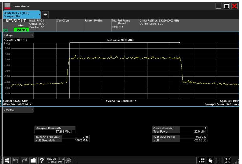
100MHz_30kHz_3625MHz_CP-OFDM QPSK_RB273@0
