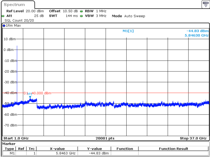
10MHz_15kHz_3555MHz_DFT-s-OFDM QPSK_RB1@0 -44.83 dBm
