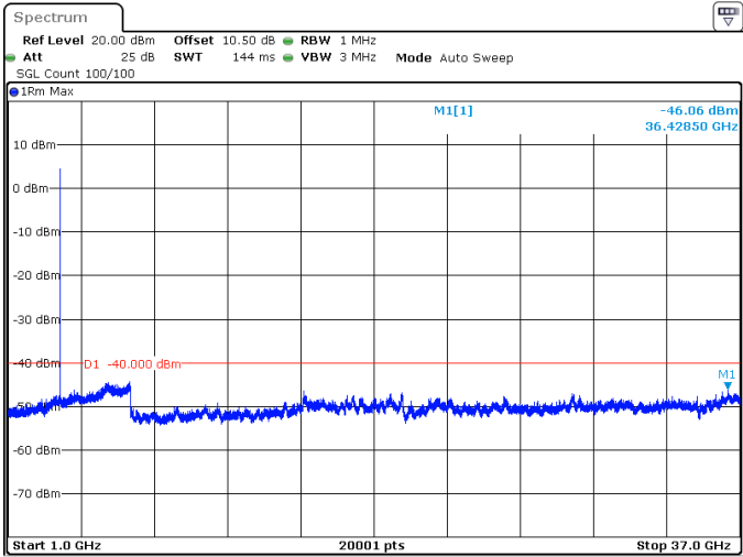
10MHz_15kHz_3555MHz_DFT-s-OFDM QPSK_RB50@0 -46.06 dBm
