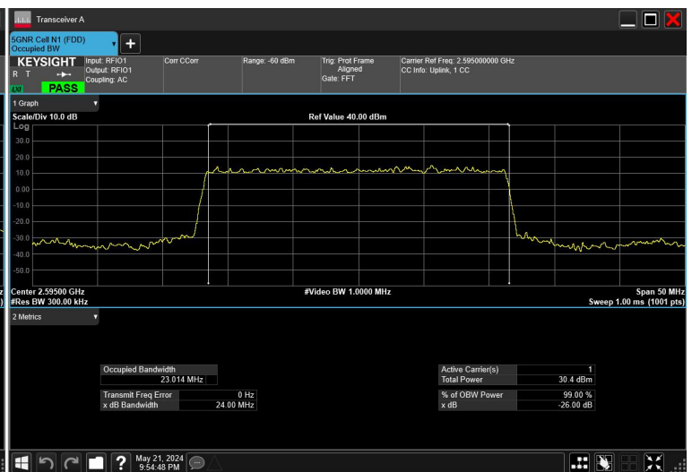
25MHz_30kHz_2595MHz_DFT-s-OFDM \pi/2 BPSK_RB64@0
