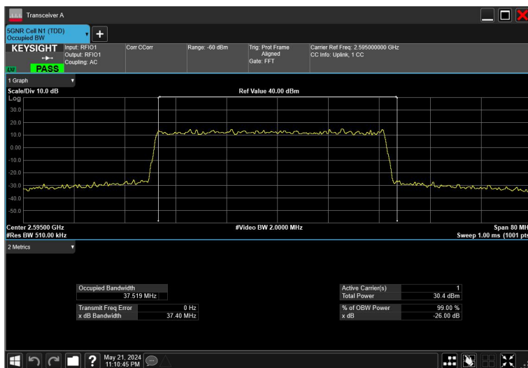
40MHz_30kHz_2595MHz_DFT-s-OFDM QPSK_RB100@0
