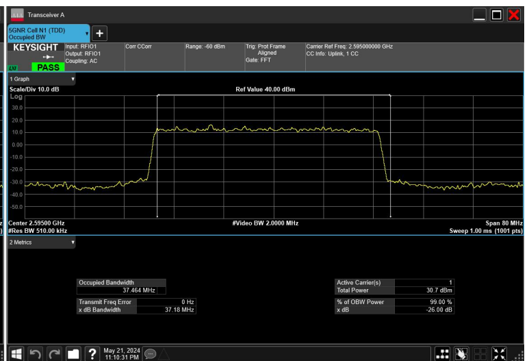
40MHz_30kHz_2595MHz_DFT-s-OFDM \pi/2 BPSK_RB100@0
