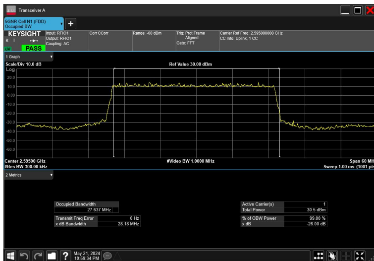
30MHz_30kHz_2595MHz_DFT-s-OFDM \pi/2 BPSK_RB75@0
