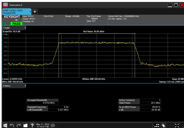
10MHz_30kHz_2592.99MHz_DFT-s-OFDM \pi/2 BPSK_RB24@0
