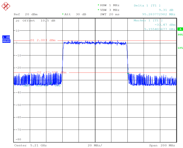
ax80_5210MHz_RU_996/67_Chain 1 95.284 MHz
