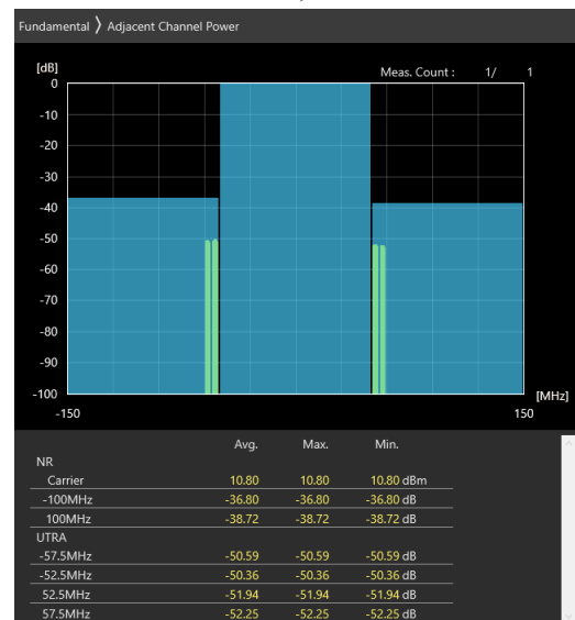
100MHz_30kHz_3600MHz_DFT-s-OFDM \pi/2 BPSK_RB135@67 -36.8 dB,-38.72 dB
