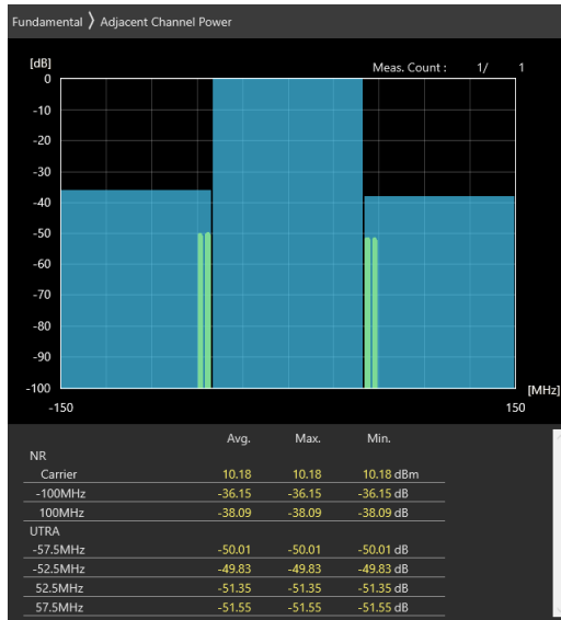
100MHz_30kHz_3600MHz_DFT-s-OFDM \pi/2 BPSK_RB270@0 -36.15 dB,-38.09 dB
