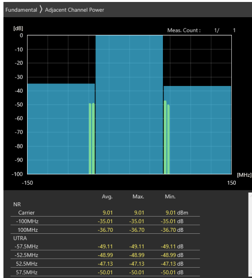
100MHz_30kHz_3650MHz_DFT-s-OFDM QPSK_RB1@272 -35.01 dB,-36.7 dB
