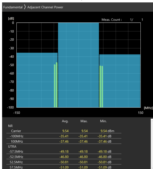
100MHz_30kHz_3600MHz_DFT-s-OFDM \pi/2 BPSK_RB1@0 -35.41 dB,-37.46 dB
