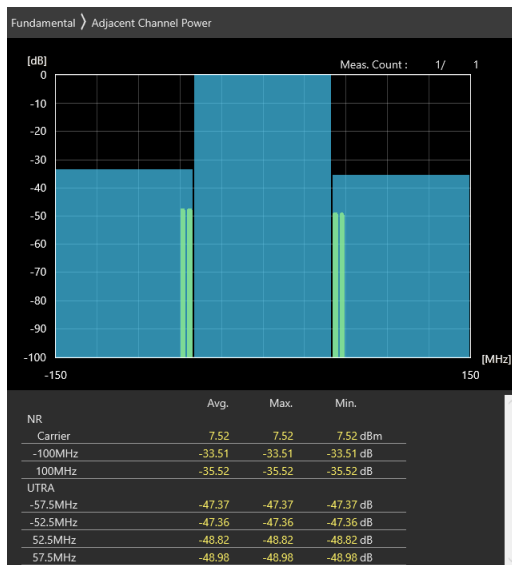
100MHz_30kHz_3650MHz_CP-OFDM QPSK_RB273@0 -33.51 dB,-35.52 dB
