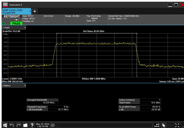
20MHz_30kHz_3500MHz_DFT-s-OFDM 256QAM_RB50@0
