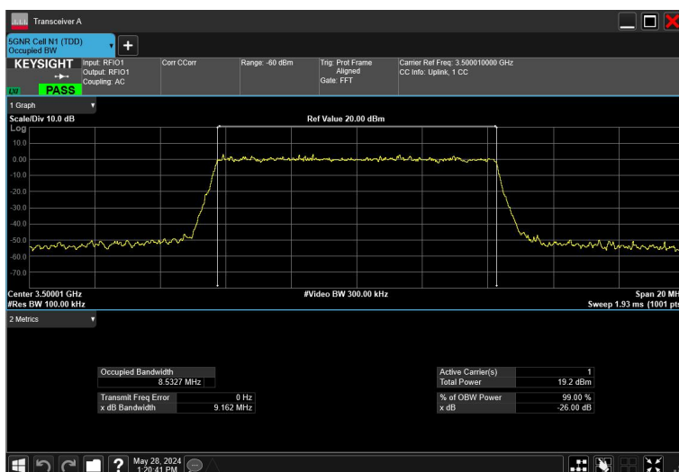
10MHz_30kHz_3500MHz_DFT-s-OFDM QPSK_RB24@0
