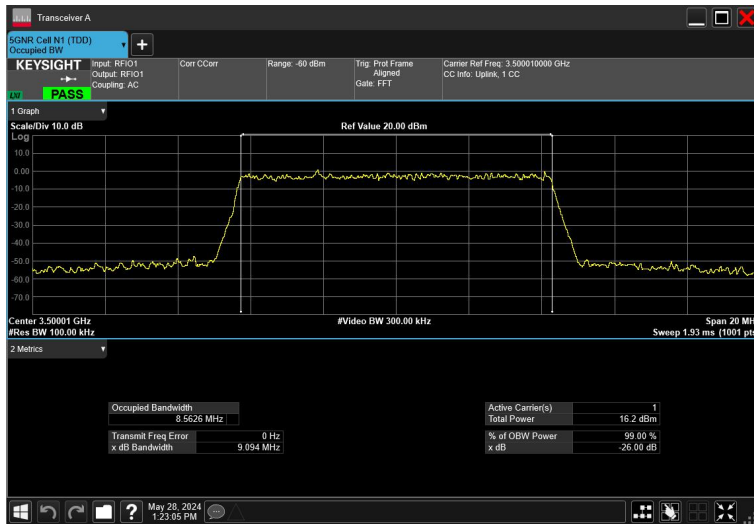
10MHz_30kHz_3500MHz_CP-OFDM QPSK_RB24@0
