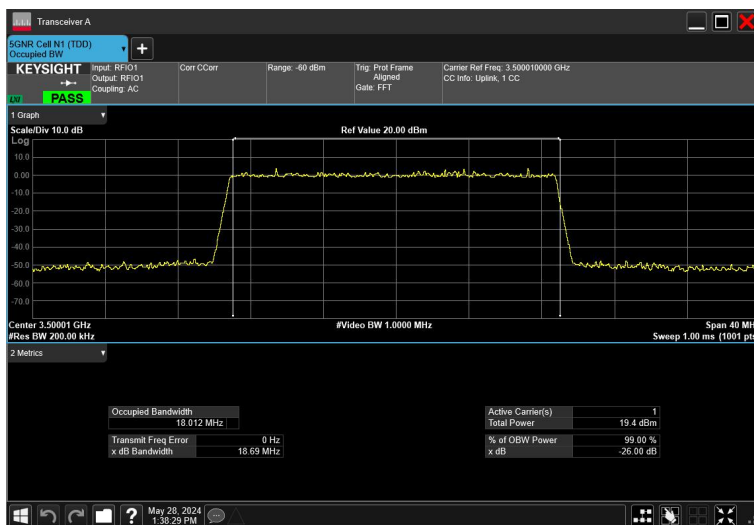
20MHz_30kHz_3500MHz_DFT-s-OFDM QPSK_RB50@0
