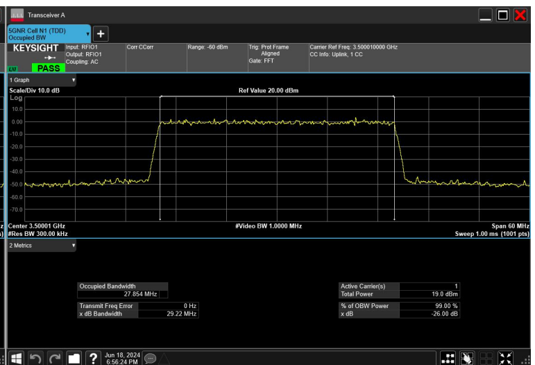
30MHz_30kHz_3500MHz_CP-OFDM QPSK_RB78@0
