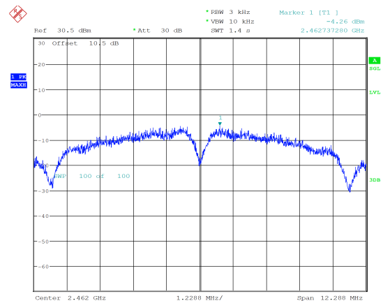
b_2462MHz_Chain 1 -4.26 dBm/3kHz
