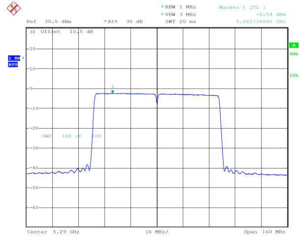
ac80_5290MHz_Chain 1 -2.54 dBm
