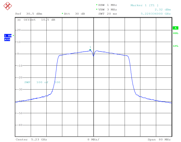
n40_5230MHz_Chain 1 2.32 dBm
