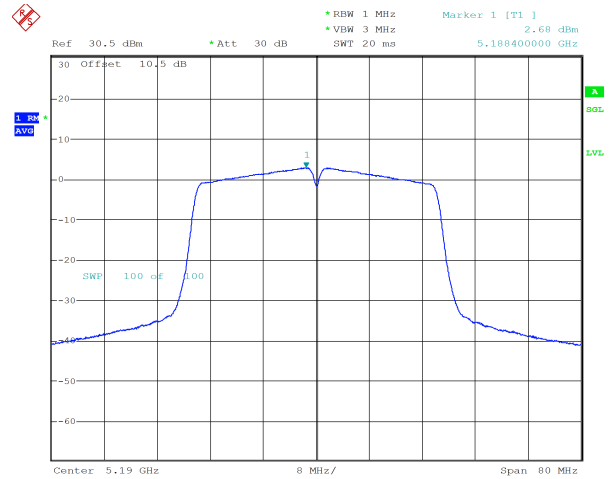
n40_5190MHz_Chain 1 2.68 dBm
