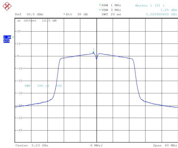
n40_5230MHz_Chain 0 1.85 dBm
