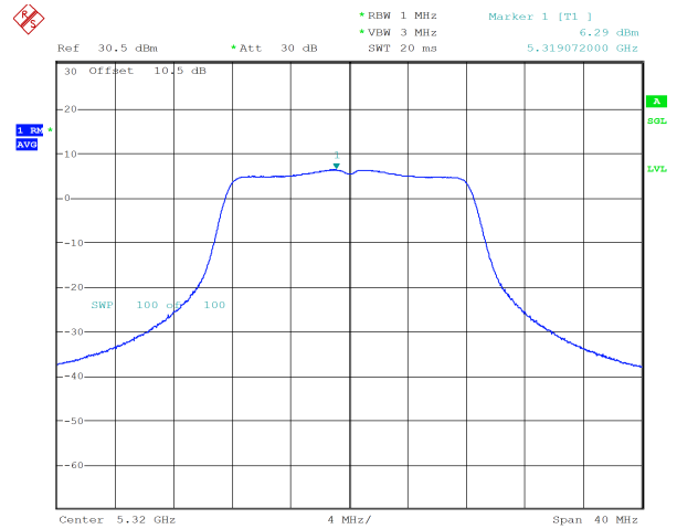
a_5320MHz_Chain 1 6.29 dBm
