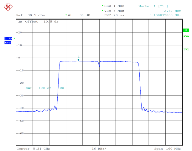
ac80_5210MHz_Chain 1 -2.67 dBm
