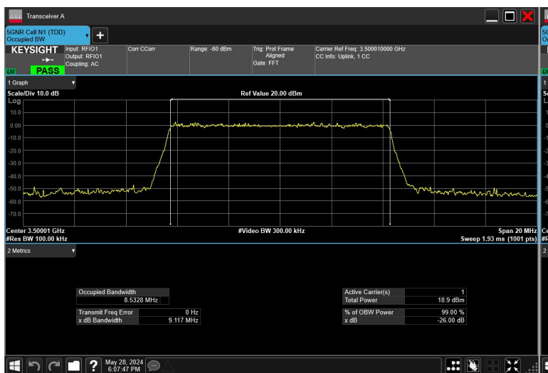
10MHz_30kHz_3500MHz_DFT-s-OFDM QPSK_RB24@0
