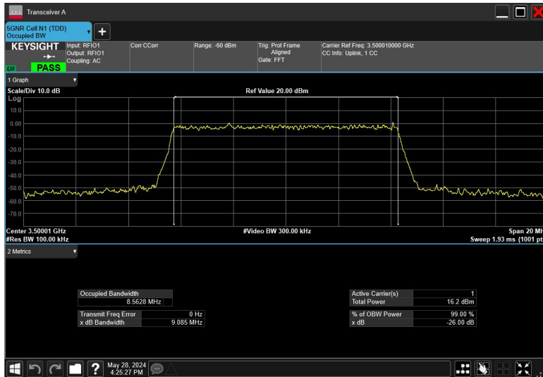
10MHz_30kHz_3500MHz_CP-OFDM QPSK_RB24@0
