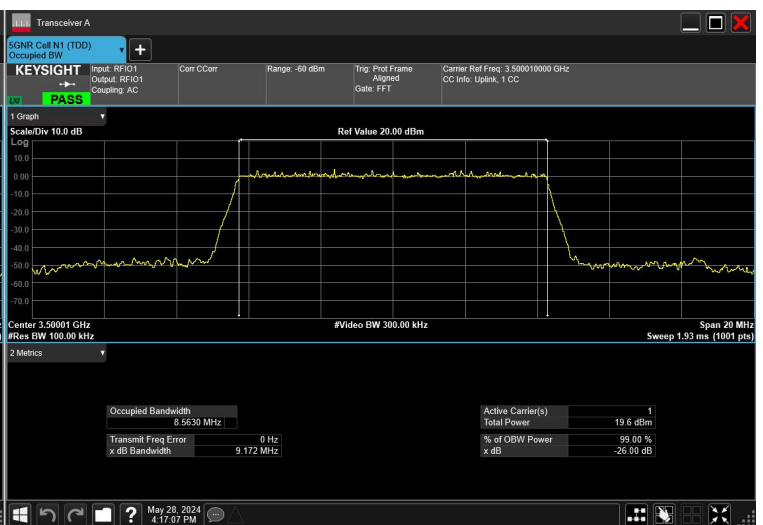
10MHz_30kHz_3500MHz_DFT-s-OFDM \pi/2 BPSK_RB24@0
