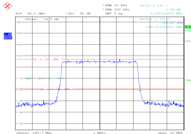
26dB Bandwidth 4.855MHz
