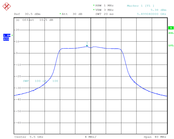
a_5500MHz_Chain 0 5.38 dBm
