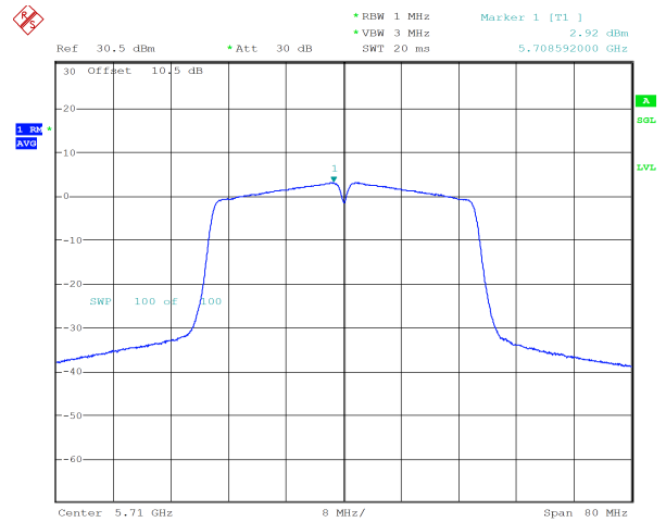
n40_5710MHz_Chain 1 2.92 dBm
