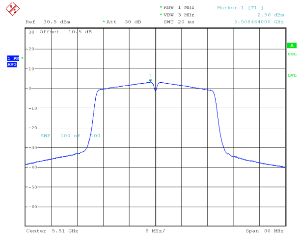
n40_5510MHz_Chain 1 2.96 dBm
