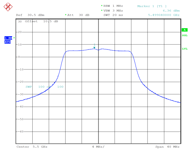
a_5500MHz_Chain 1 6.36 dBm
