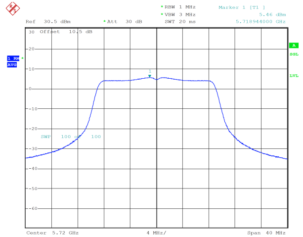
n20_5720MHz_Chain 1 5.46 dBm
