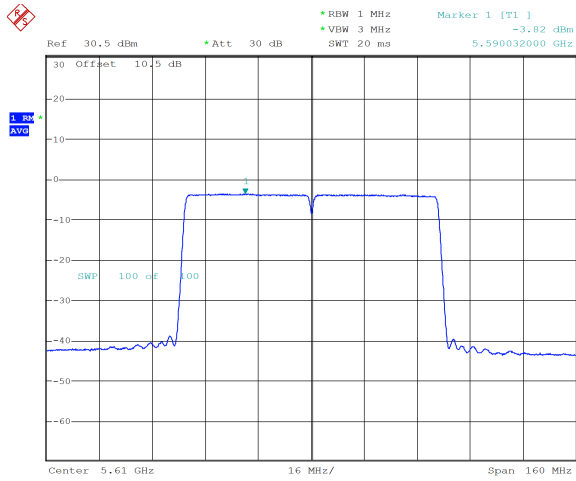
ac80_5610MHz_Chain 0 -3.82 dBm
