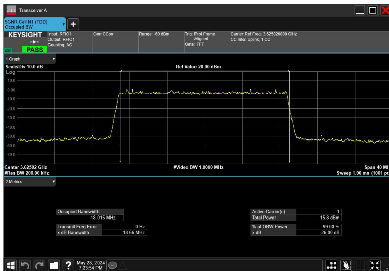
20MHz_30kHz_3625MHz_DFT-s-OFDM 256QAM_RB50@0
