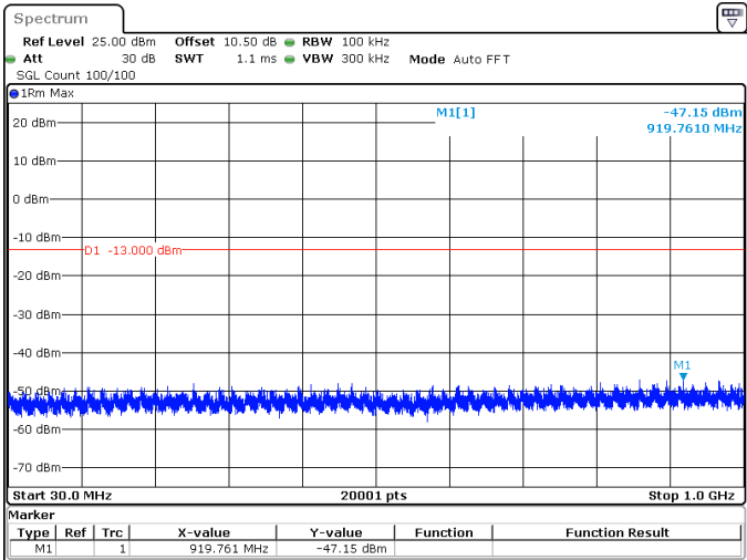
80MHz_30kHz_3490MHz_DFT-s-OFDM QPSK_RB1@0 -47.15 dBm
