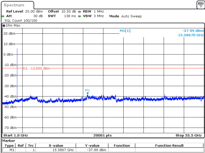
30MHz_30kHz_3535MHz_DFT-s-OFDM QPSK_RB1@0 -37.99 dBm
