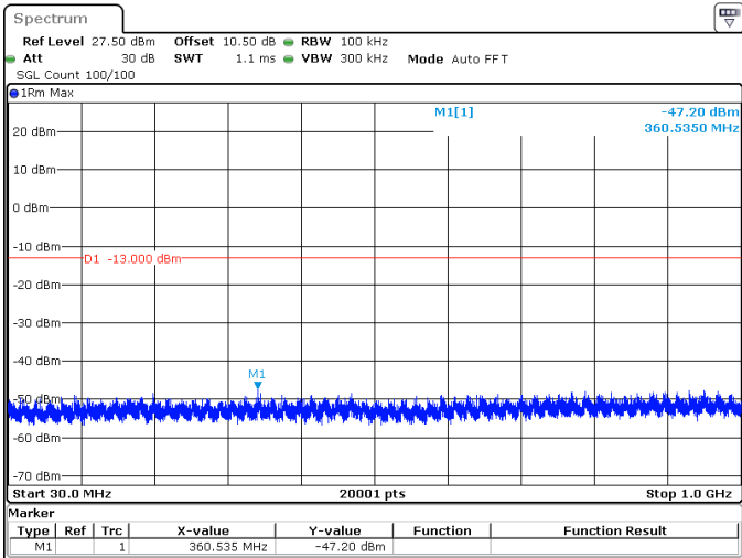
25MHz_30kHz_3500MHz_DFT-s-OFDM QPSK_RB1@0 -47.20 dBm
