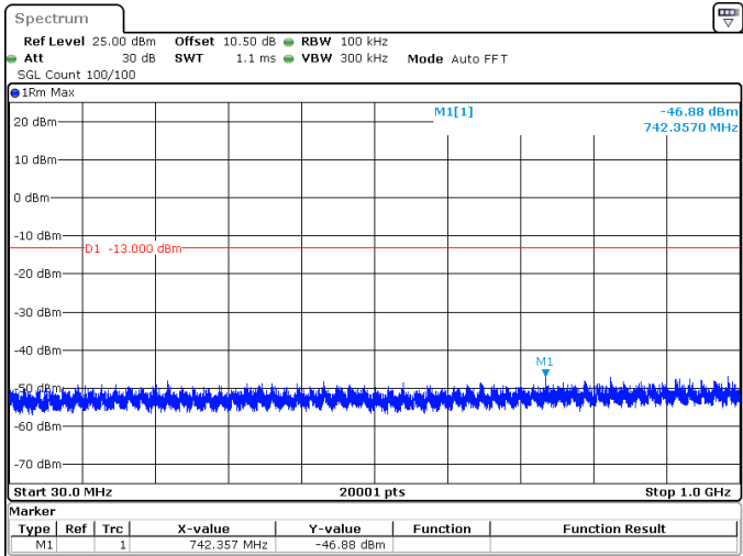
100MHz_30kHz_3500MHz_DFT-s-OFDM QPSK_RB1@0 -46.88 dBm
