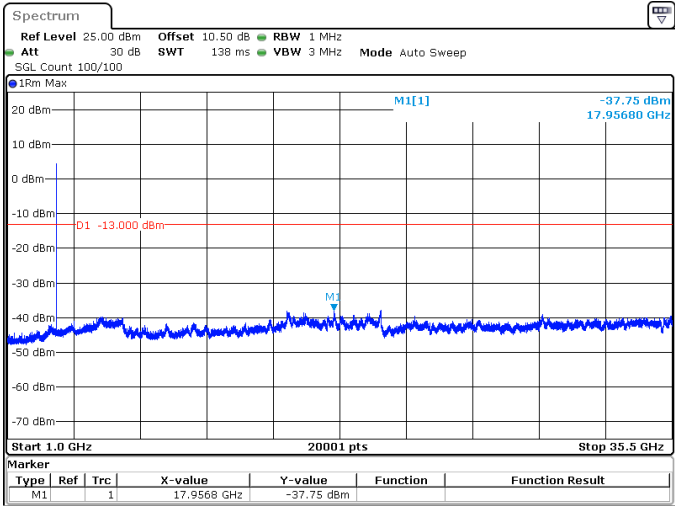
80MHz_30kHz_3490MHz_DFT-s-OFDM QPSK_RB1@216 -37.75 dBm
