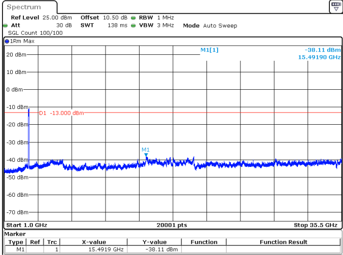
100MHz_30kHz_3500MHz_DFT-s-OFDM QPSK_RB270@0 -38.11 dBm
