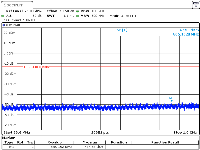
80MHz_30kHz_3490MHz_DFT-s-OFDM QPSK_RB216@0 -47.33 dBm
