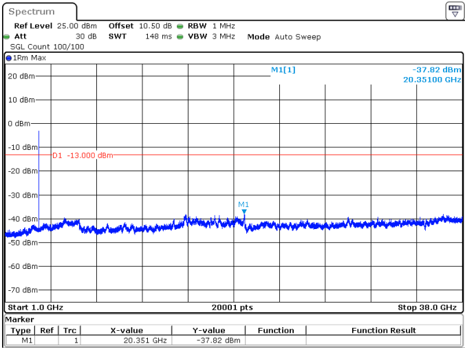
15MHz_15kHz_3707.5MHz_DFT-s-OFDM QPSK_RB75@0 -37.82 dBm
