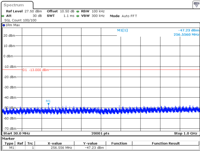
25MHz_30kHz_3500MHz_DFT-s-OFDM QPSK_RB64@0 -47.23 dBm
