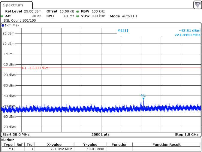
40MHz_30kHz_3470MHz_DFT-s-OFDM QPSK_RB1@0 -43.81 dBm
