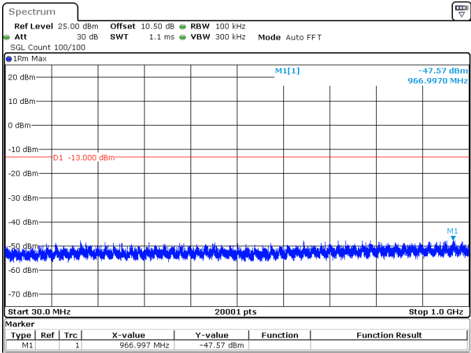
30MHz_30kHz_3535MHz_DFT-s-OFDM QPSK_RB75@0 -47.57 dBm
