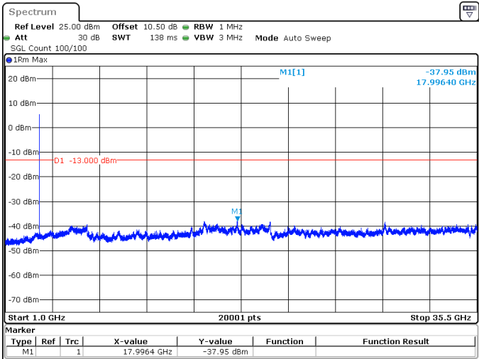
30MHz_30kHz_3500MHz_DFT-s-OFDM QPSK_RB1@0 -37.95 dBm
