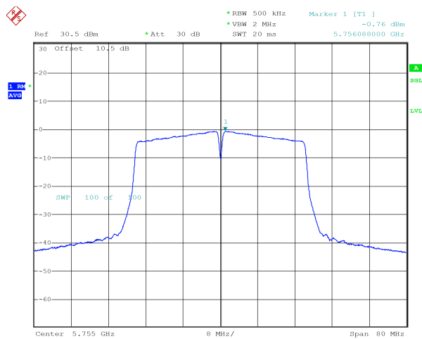
n40_5755MHz_Chain 0 -0.76 dBm
