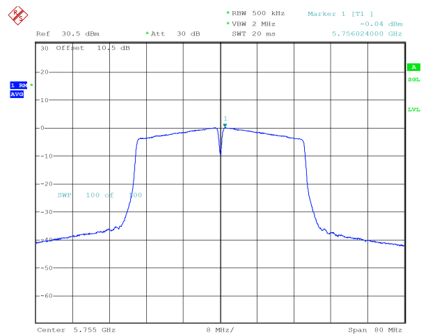
n40_5755MHz_Chain 1 -0.04 dBm
