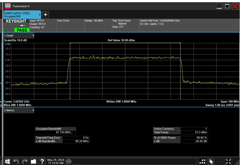
90MHz_30kHz_3625MHz_CP-OFDM QPSK_RB245@0
