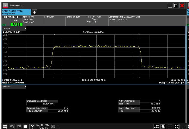
60MHz_30kHz_3625MHz_DFT-s-OFDM QPSK_RB162@0
