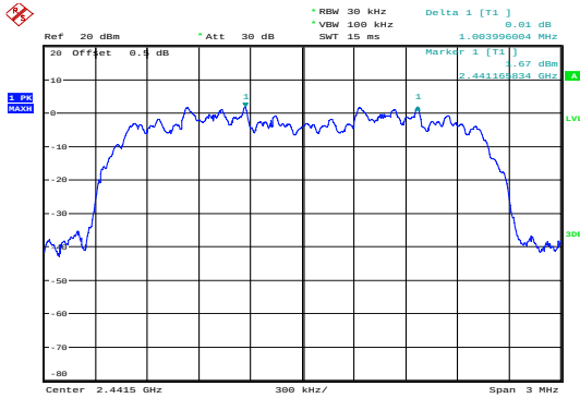
\pi/4 -DQPSK_Middle 1.004MHz
