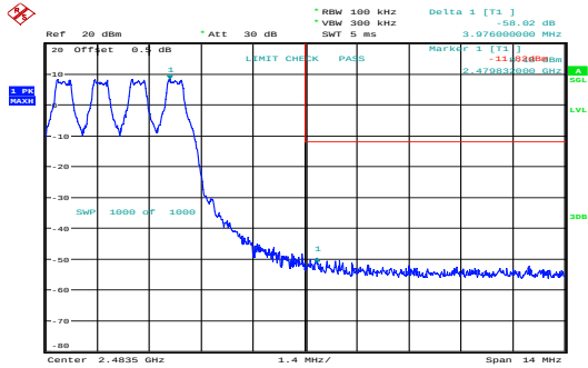
GFSK_Hopping_Upper
