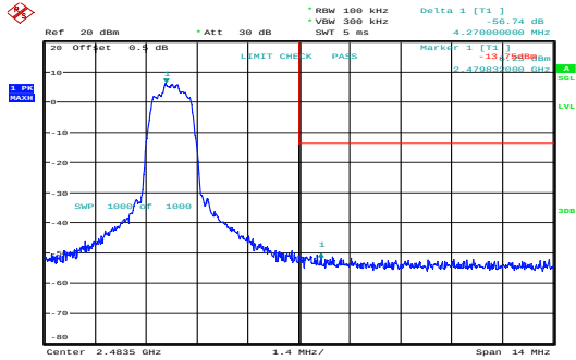
\pi/4 -DQPSK_High
