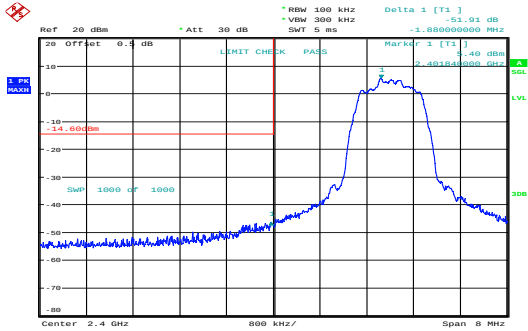
\pi/4 -DQPSK_Low
