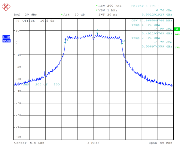
n20_5500MHz_Chain 1 17.869 MHz
