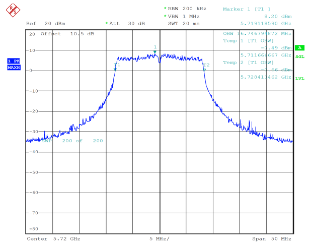
a_5720MHz_Chain 1 16.747 MHz
