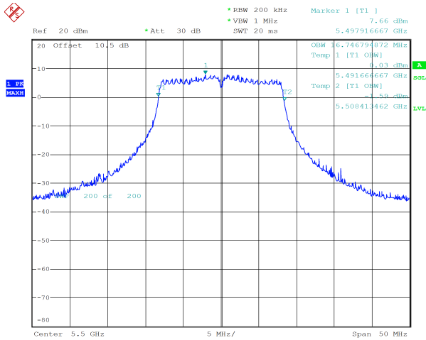
a_5500MHz_Chain 1 16.747 MHz
