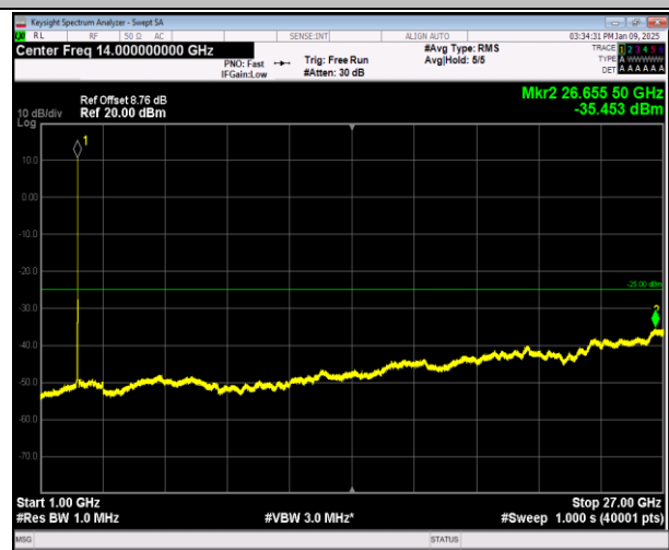
7-7-10MHz-20MHz-QPSK-QPSK-21206-21350-50RB#0-100RB#0-1000~27000MHz-PASS
