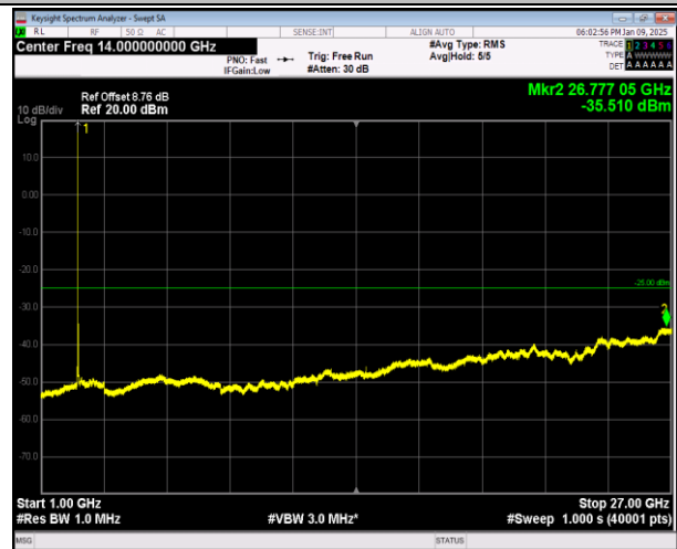
7-7-20MHz-20MHz-QPSK-QPSK-21001-21199-1RB#0-ORB #0-1000~27000MHz-PASS
