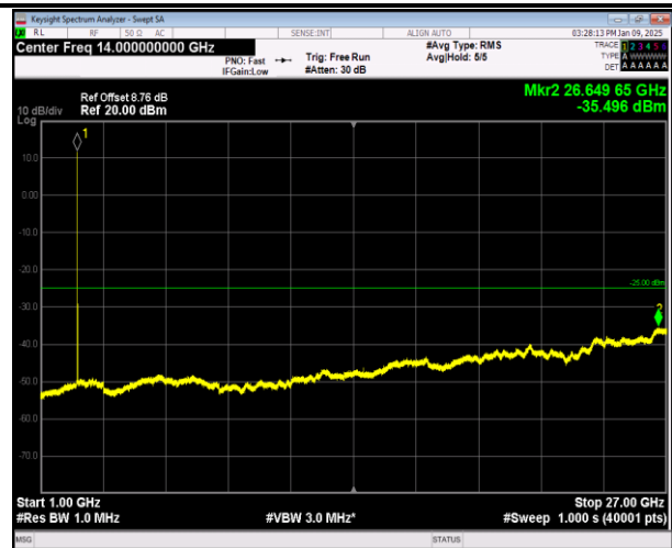
7-7-10MHz-20MHz-QPSK-QPSK-21006-21150-1RB#0-1RB #99-1000~27000MHz-PASS
