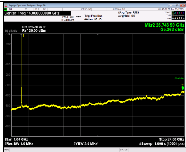
7-7-20MHz-10MHz-QPSK-QPSK-20850-20994-1RB#0-0RB #0-1000~27000MHz-PASS
