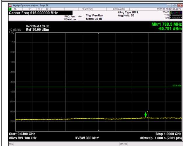
7-7-10MHz-20MHz-QPSK-QPSK-21006-21150-50RB#0-1 00RB#0-30~1000MHz-PASS
