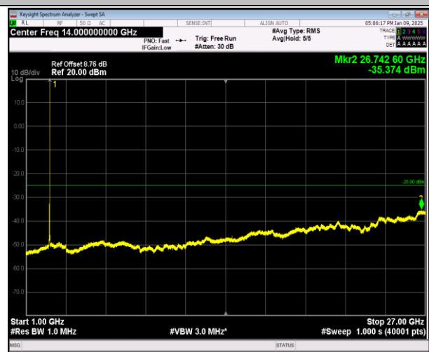
7-7-20MHz-10MHz-QPSK-QPSK-21051-21195-1RB#99-0R B#0-1000~27000MHz-PASS
