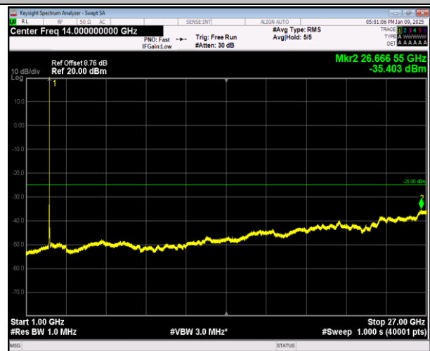
7-7-20MHz-10MHz-QPSK-QPSK-20850-20994-1RB#99-0R B#0-1000~27000MHz-PASS
