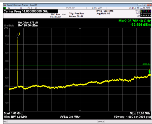
7-7-20MHz-10MHz-QPSK-QPSK-21251-21395-100RB#0-5 0RB#0-1000~27000MHz-PASS
