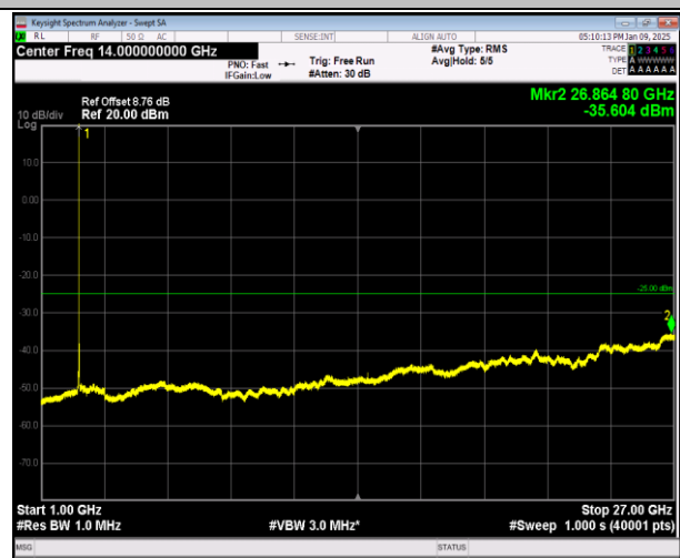
7-7-20MHz-10MHz-QPSK-QPSK-21251-21395-1RB#0-0RB #0-1000~27000MHz-PASS
