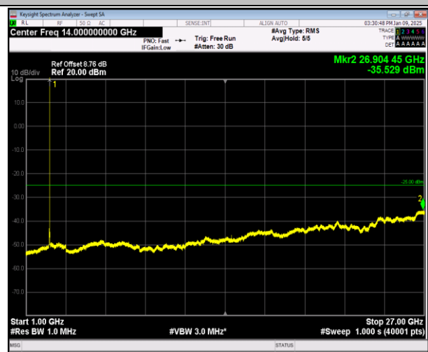
7-7-10MHz-20MHz-QPSK-QPSK-21206-21350-1RB#0-0RB #0-1000~27000MHz-PASS
