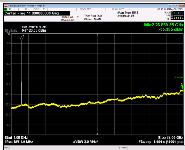
7-7-10MHz-20MHz-QPSK-QPSK-21206-21350-1RB#0-0-1RB #99-1000~27000MHz-PASS
