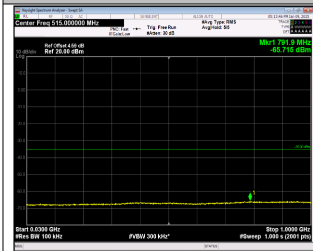
7-7-20MHz-10MHz-QPSK-QPSK-21251-21395-100RB#0-50RB#0-30~1000MHz-PASS
