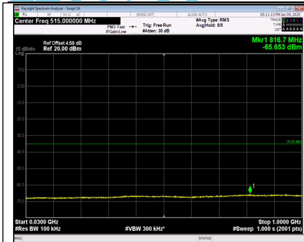
7-7-20MHz-10MHz-QPSK-QPSK-21251-21395-1RB#99-0RB#0-30~1000MHz-PASS
