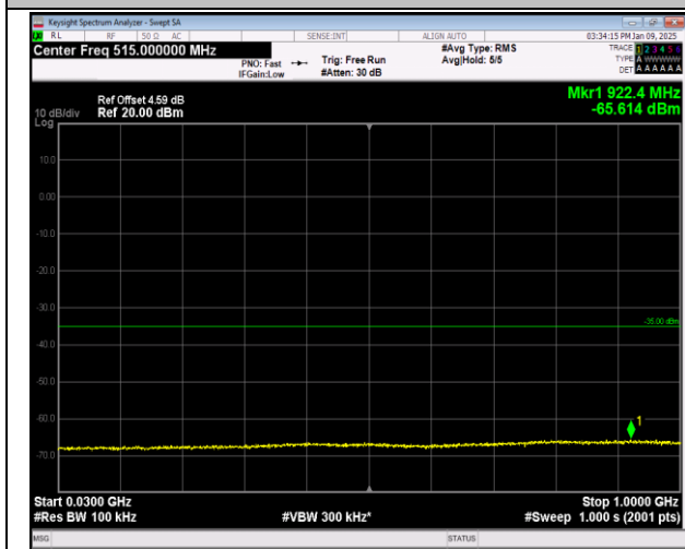
7-7-10MHz-20MHz-QPSK-QPSK-21206-21350-50RB#0-100RB#0-30~1000MHz-PASS
