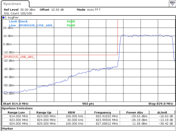
5MHz_15kHz_826.5MHz_DFT-s-OFDM QPSK_RB25@0 -26.19 dBm
