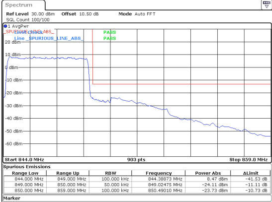
5MHz_15kHz_846.5MHz_DFT-s-OFDM QPSK_RB25@0 -23.73 dBm
