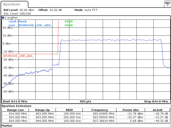
20MHz_15kHz_834MHz_DFT-s-OFDM QPSK_RB100@0 -25.57 dBm
