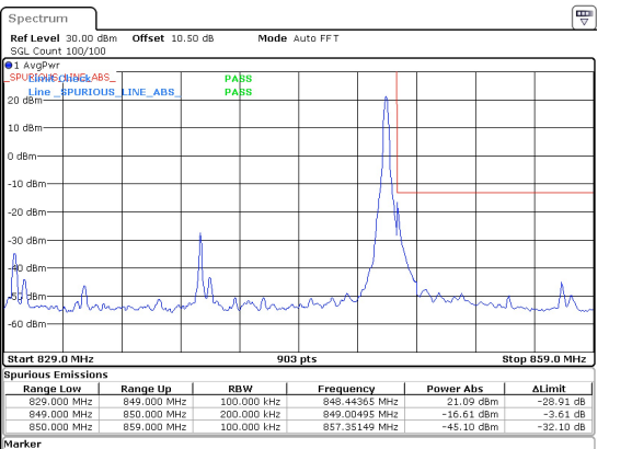
20MHz_15kHz_839MHz_DFT-s-OFDM QPSK_RB1@105 -16.61 dBm
