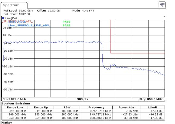
20MHz_15kHz_839MHz_DFT-s-OFDM QPSK_RB100@0 -27.23 dBm
