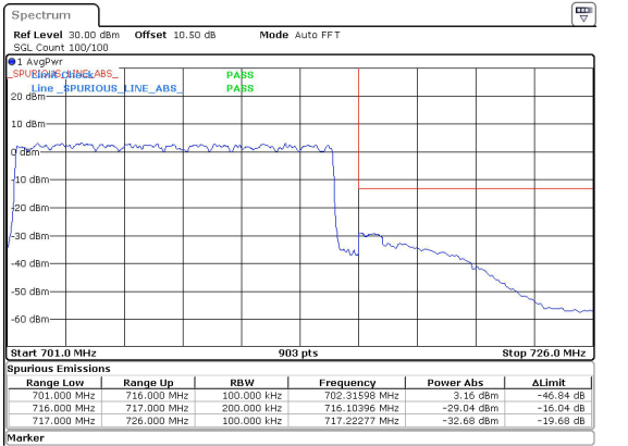
15MHz_15kHz_708.5MHz_DFT-s-OFDM QPSK_RB75@0&-29.04 dBm
