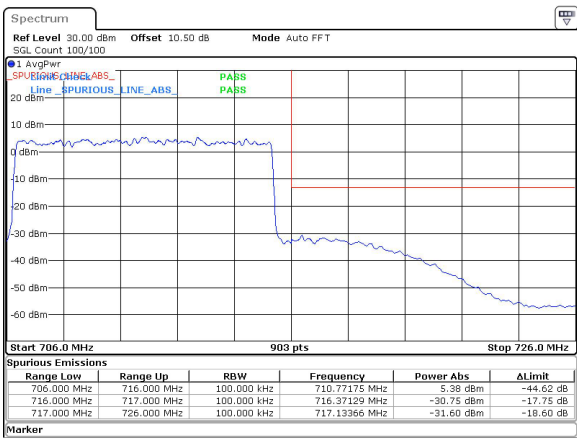
10MHz_15kHz_711MHz_DFT-s-OFDM QPSK_RB50@0&-30.75 dBm
