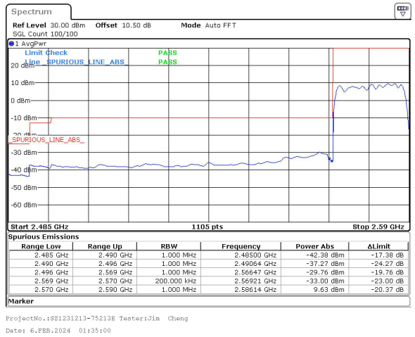
20MHz_30kHz_2580MHz_DFT-s-OFDM QPSK_RB50@0&-42.38 dBm
