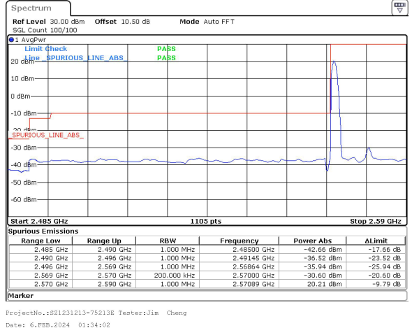
20MHz_30kHz_2580MHz_DFT-s-OFDM QPSK_RB1@0&20.21 dBm
