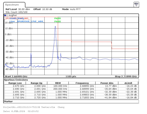
20MHz_30kHz_2679.99MHz_DFT-s-OFDM QPSK_RB1@50&13.77 dBm
