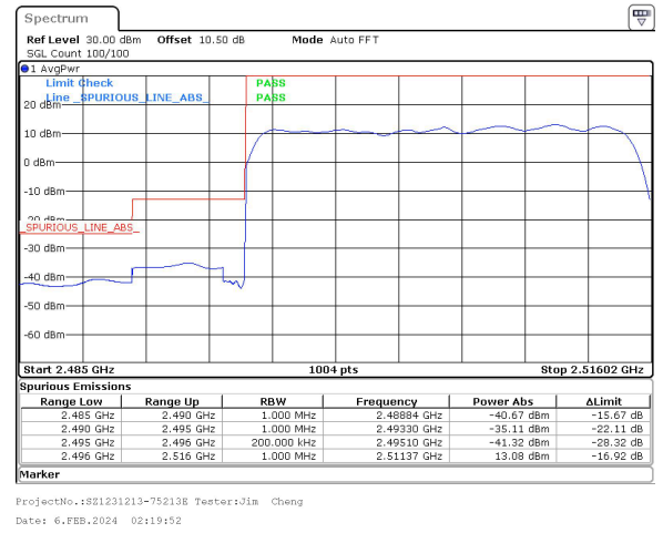
20MHz_30kHz_2506.02MHz_DFT-s-OFDM QPSK_RB50@0&-40.67 dBm
