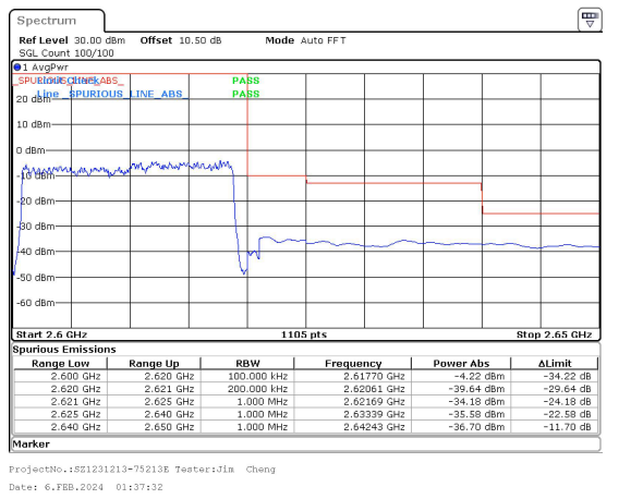
20MHz_30kHz_2610MHz_DFT-s-OFDM QPSK_RB50@0&-36.70 dBm
