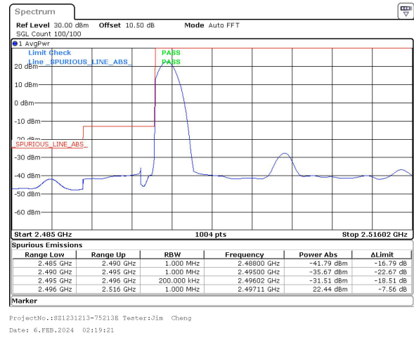
20MHz_30kHz_2506.02MHz_DFT-s-OFDM QPSK_RB1@0&22.44 dBm
