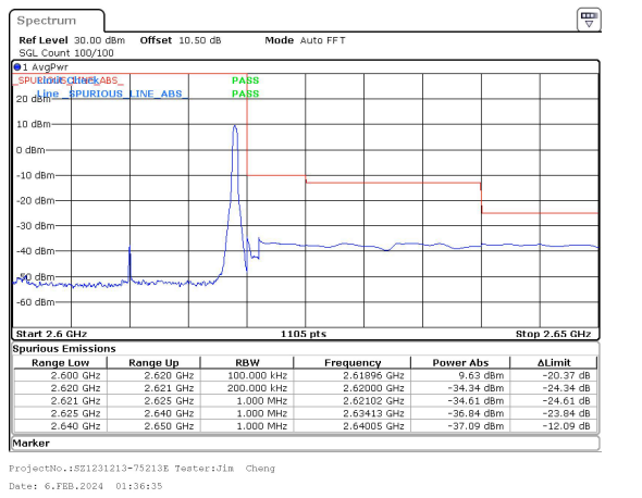
20MHz_30kHz_2610MHz_DFT-s-OFDM QPSK_RB1@50&-37.09 dBm
