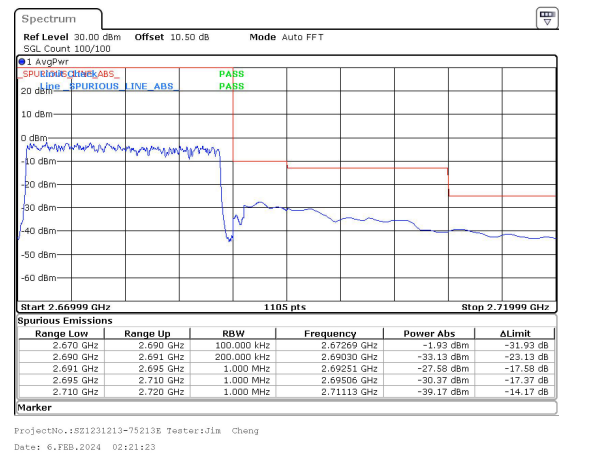
20MHz_30kHz_2679.99MHz_DFT-s-OFDM QPSK_RB50@0&-39.17 dBm
