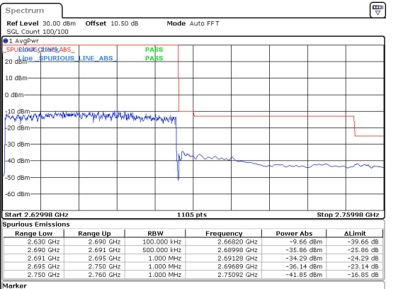
60MHz_30kHz_2659.98MHz_DFT-s-OFDM QPSK_RB162@0&-41.85 dBm
