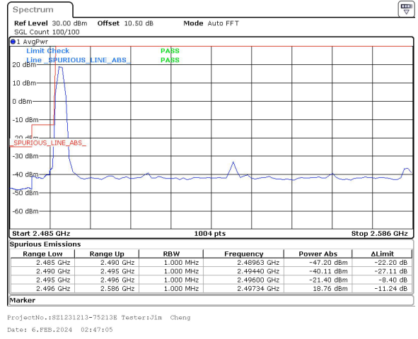
90MHz_30kHz_2541MHz_DFT-s-OFDM QPSK_RB1@0&-21.40 dBm
