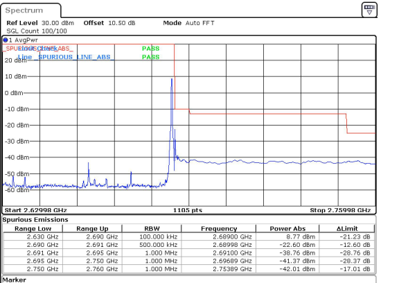
60MHz_30kHz_2659.98MHz_DFT-s-OFDM QPSK_RB1@161&-22.60 dBm
