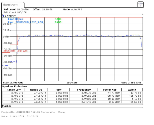
90MHz_30kHz_2541MHz_DFT-s-OFDM QPSK_RB243@0&-18.10 dBm
