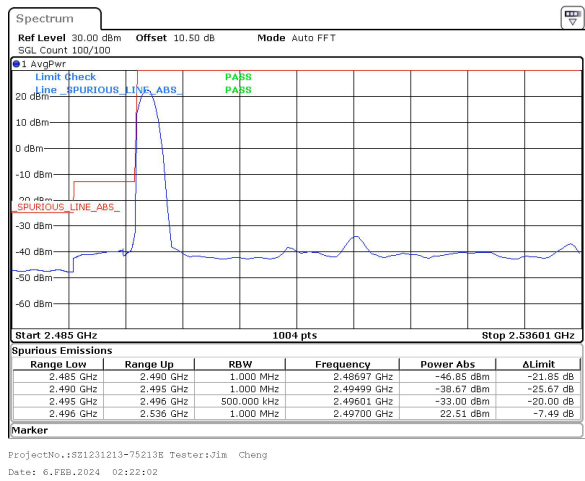
40MHz_30kHz_2516.01MHz_DFT-s-OFDM QPSK_RB1@0&22.51 dBm
