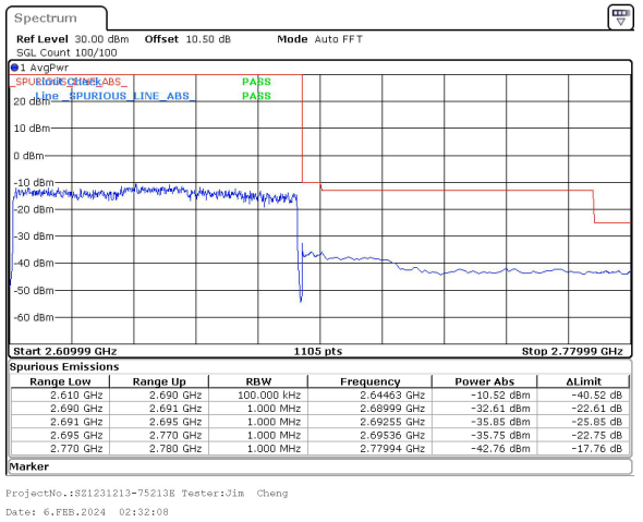
80MHz_30kHz_2649.99MHz_DFT-s-OFDM QPSK_RB216@0&-42.76 dBm
