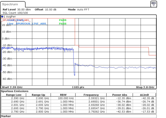
100MHz_30kHz_2640MHz_DFT-s-OFDM QPSK_RB270@0&-42.53 dBm
