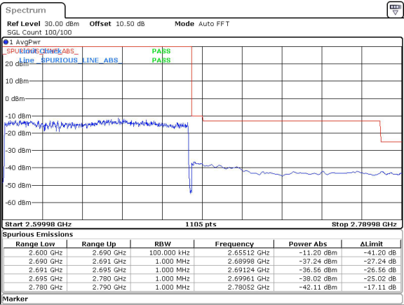
90MHz_30kHz_2644.98MHz_DFT-s-OFDM QPSK_RB243@0&-42.11 dBm
