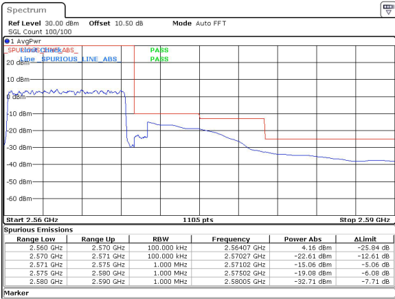
10MHz_15kHz_2565MHz_DFT-s-OFDM QPSK_RB50@0&-15.06 dBm
