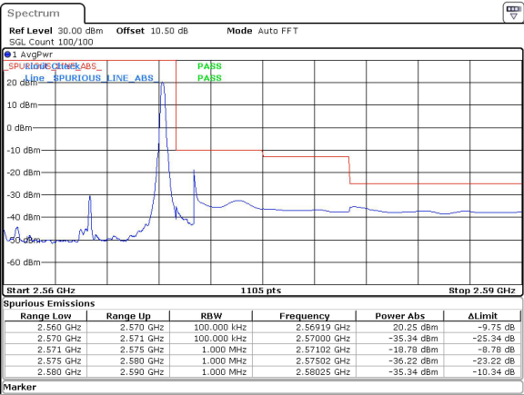
10MHz_15kHz_2565MHz_DFT-s-OFDM QPSK_RB1@51&-18.78 dBm
