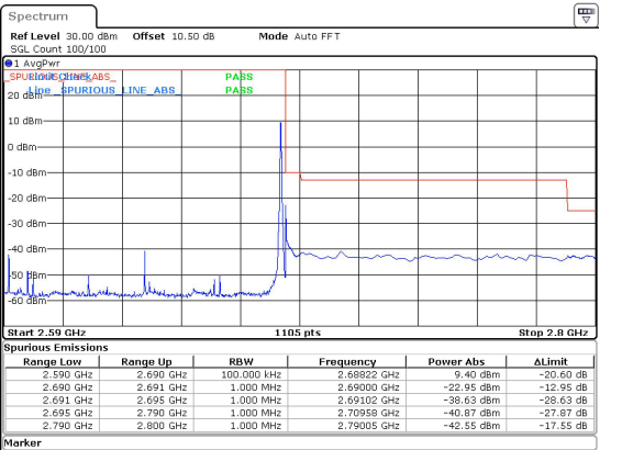
100MHz_30kHz_2640MHz_DFT-s-OFDM QPSK_RB1@272&-22.95 dBm
